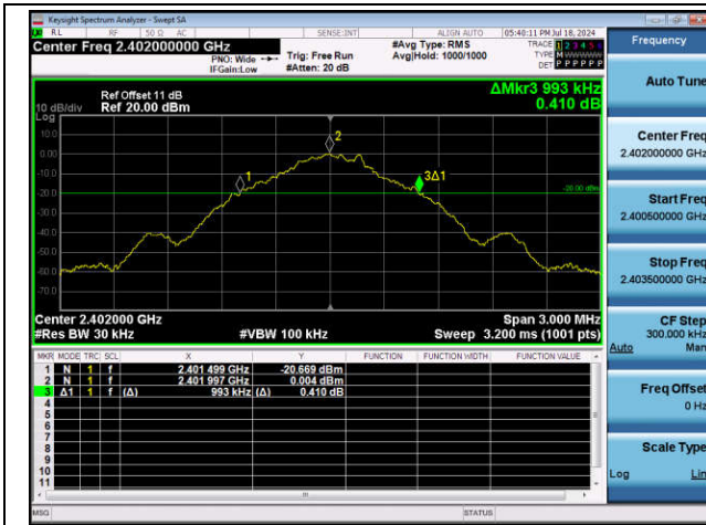
DH5-Ant1-2402
