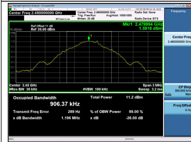
DH5-Ant1-2480
