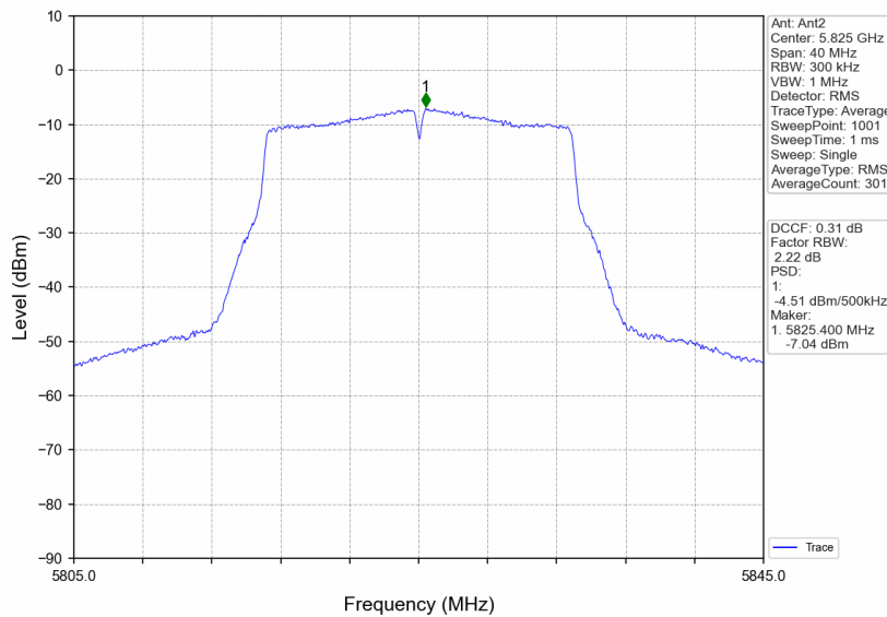
802.11n(HT20)_HCH_5825MHz_Ant2_NTNV
