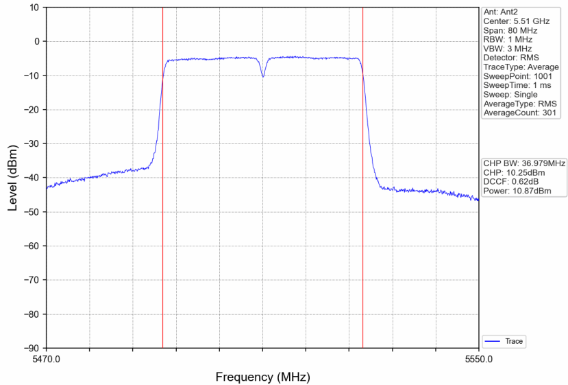
802.11n(HT40)_LCH_5510MHz_Ant2_NTNV
