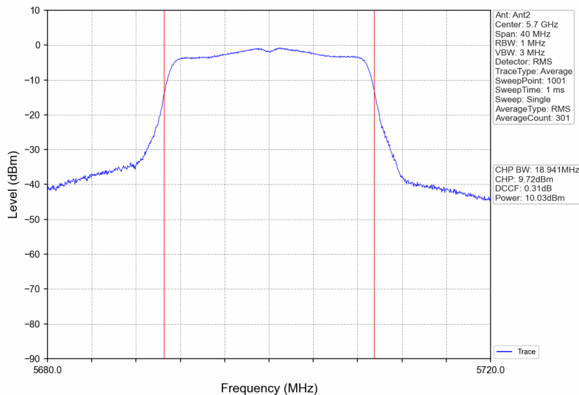
802.11n(HT20)_HCH_5700MHz_Ant2_NTNV
