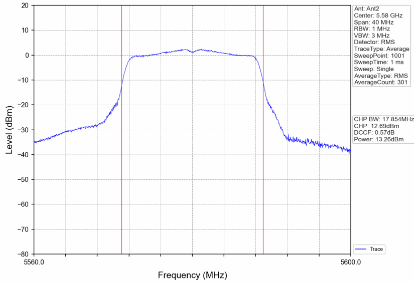
802.11a_MCH_5580MHz_Ant2_NTNV
