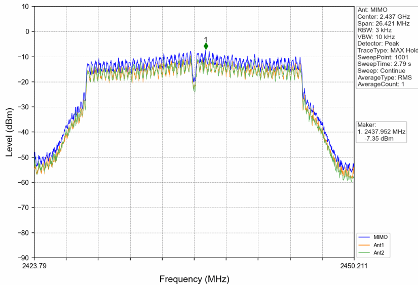
802.11n(HT20)_MCH_2437MHz_MIMO_NTNV
