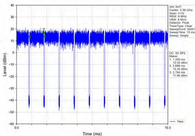
802.11a_MCH_5580MHz_Ant1_NTNV
