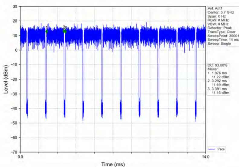
802.11ac(VHT20)_HCH_5700MHz_Ant1_NTNV
