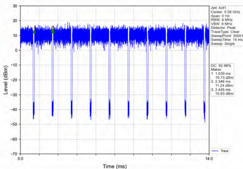
802.11n(HT20) MCH 5580MHz Ant1 NTV
