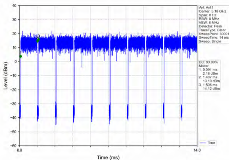
802.11ac(VHT20) LCH 5180MHz Ant1 NTNV
