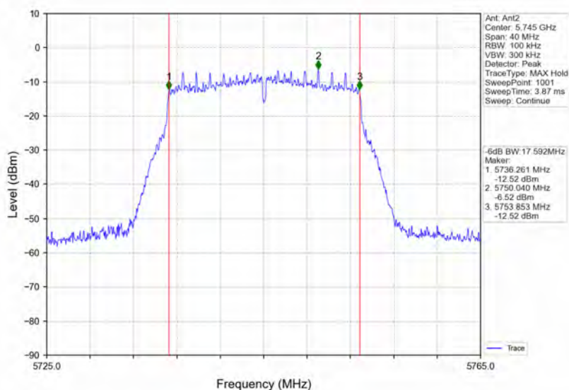
802.11n(HT20) LCH_5745MHz_Ant2_NTNV
