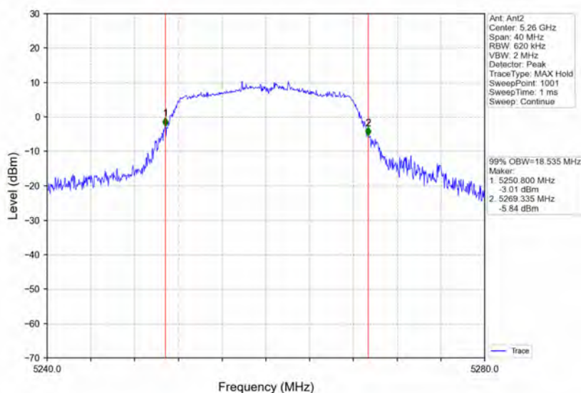
802.11a LCH_5260MHz_Ant2_NTNV
