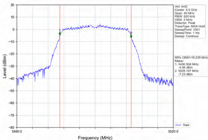
802.11n(HT20) LCH_5500MHz_Ant2_NTNV
