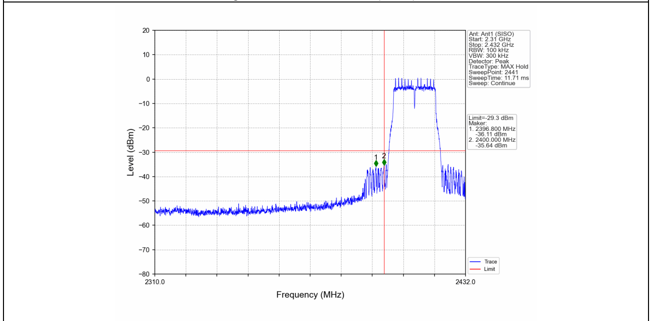
802.11g_LCH_2412MHz_Ant1 (SISO)_NTNV
