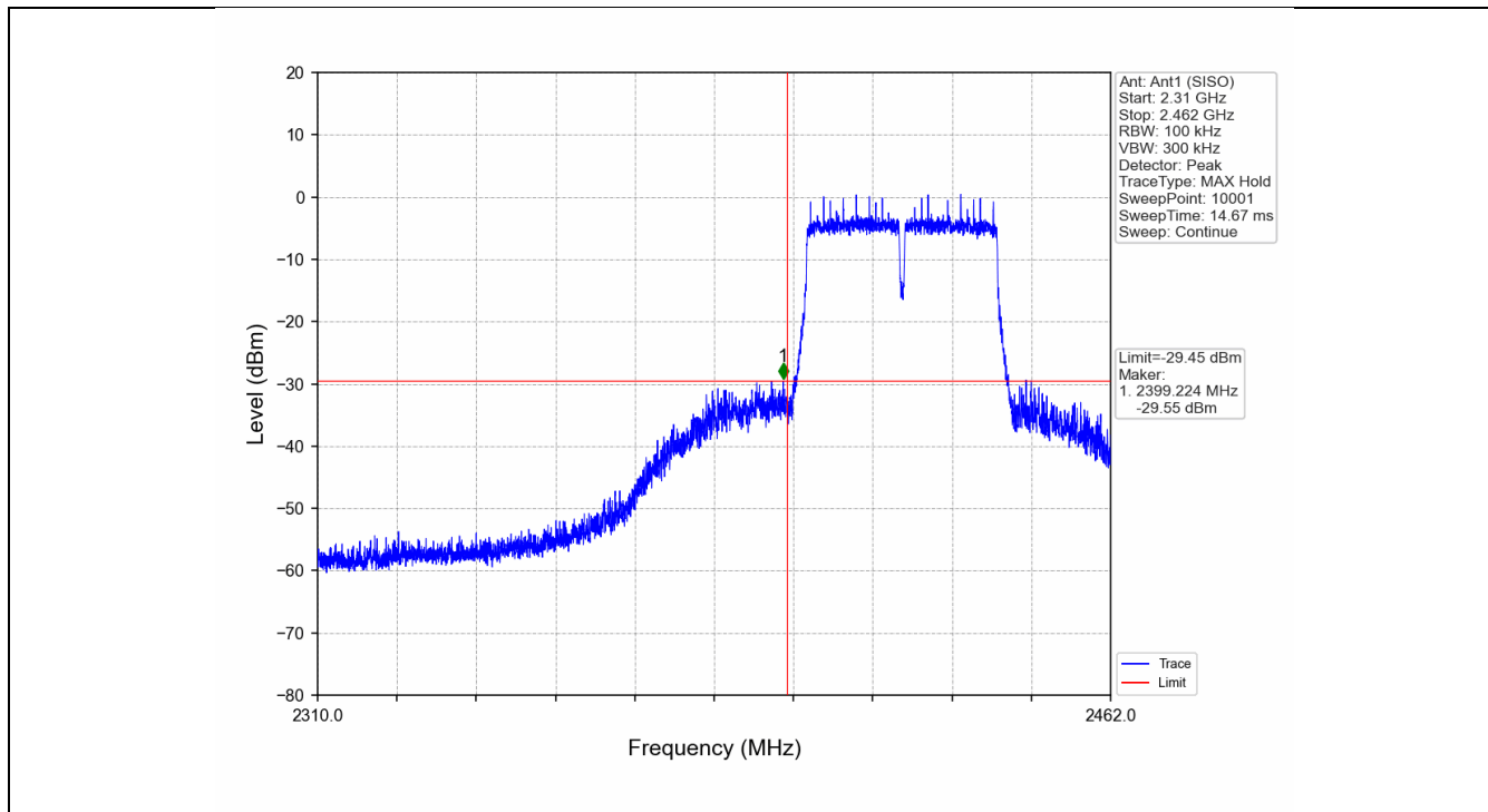
802.11n(HT40)_LCH_2422MHz_Ant1 (SISO)_NTNV
