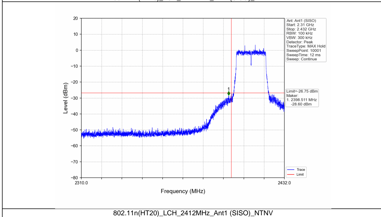
802.11n(HT20)_LCH_2412MHz_Ant1 (SISO)_NTNV
