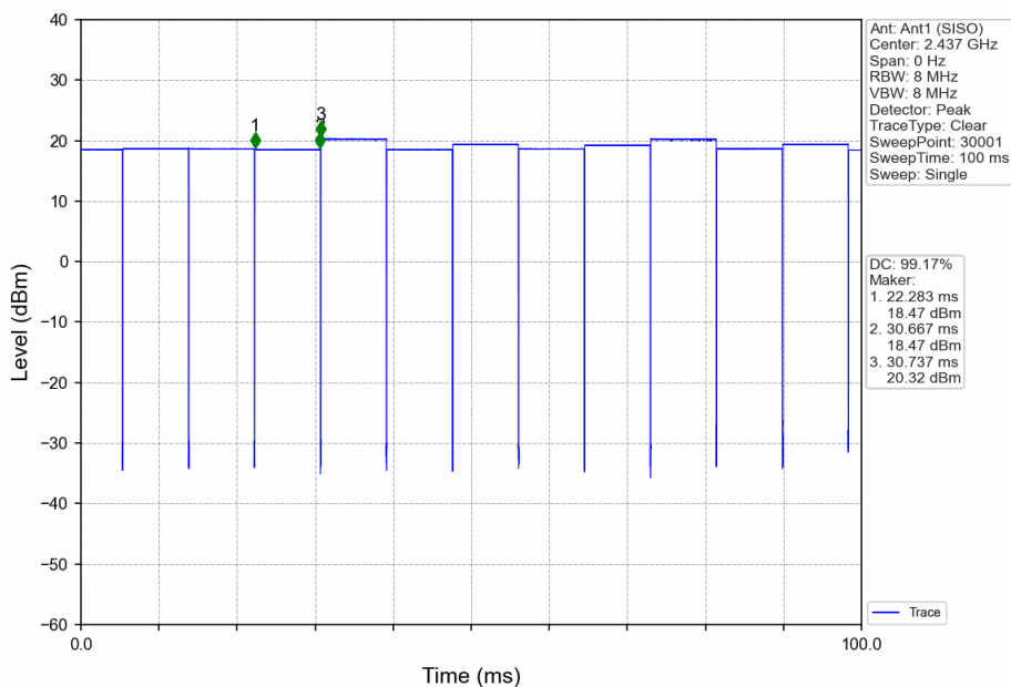
802.11b_MCH_2437MHz_Ant1 (SISO)_NTNV
