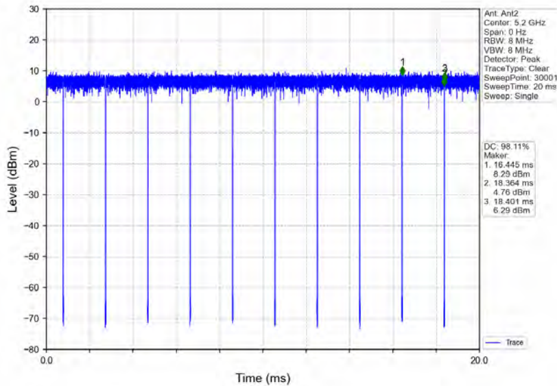
802.11n(HT20)_MCH_5200MHz_Ant2_NTNV
