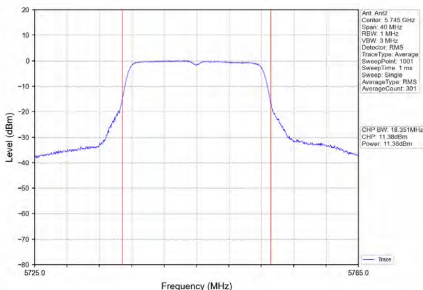
802.11a_LCH_5745MHz_Ant2_NTNV
