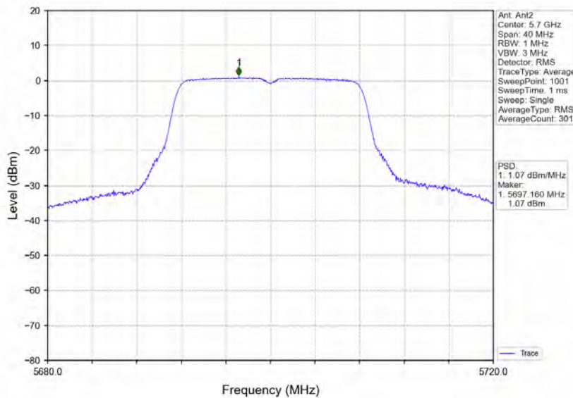
802.11a_HCH_5700MHz_Ant2_NTNV
