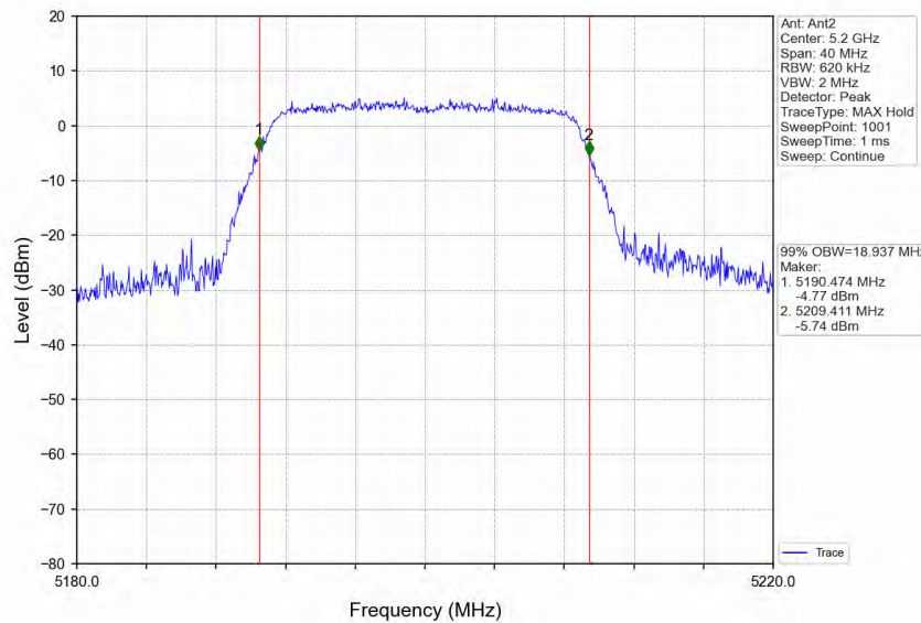
802.11n(HT20)_MCH_5200MHz_Ant2_NTNV
