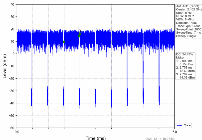
802.11n(HT20)_HCH_2462MHz_Ant1 (SISO)_NTNV
