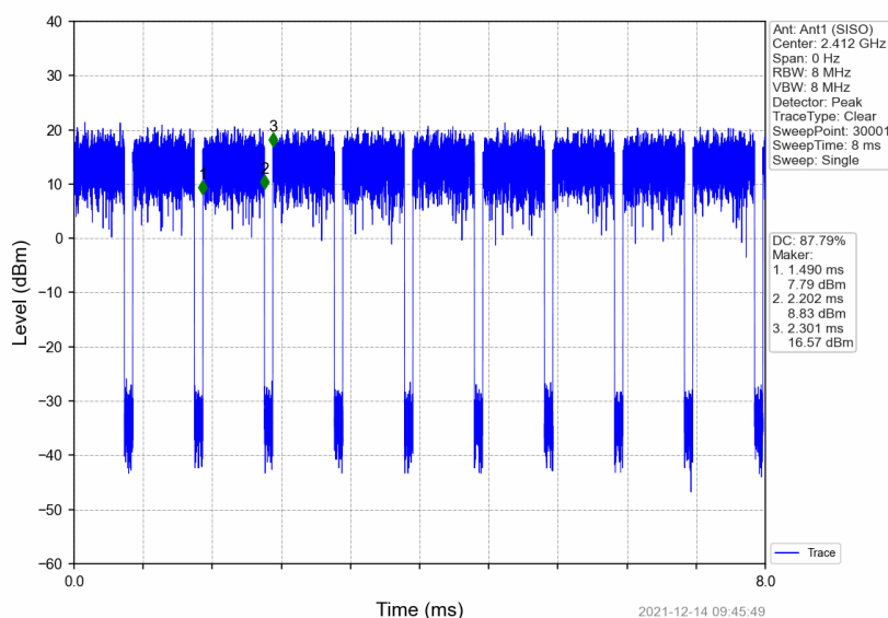
802.11g_LCH_2412MHz_Ant1 (SISO)_NTNV
