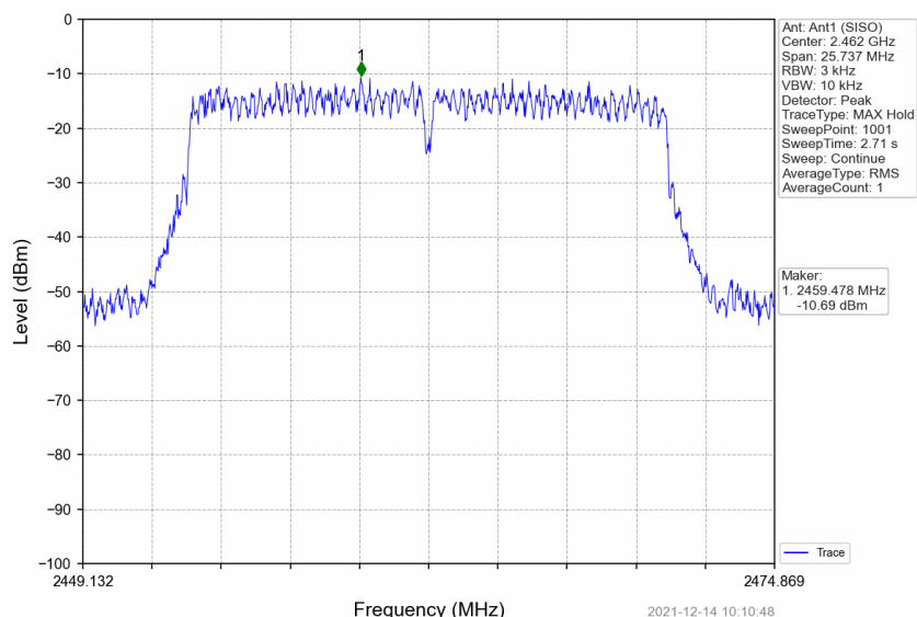
802.11n(HT20)_HCH_2462MHz_Ant1 (SISO)_NTNV
