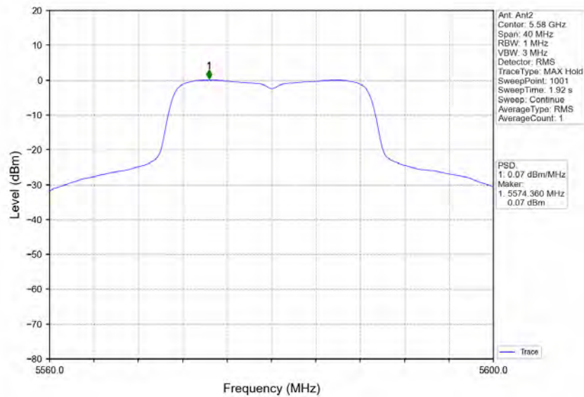
802.11n(HT20)_MCH_5580MHz_MIMO_NTNV
