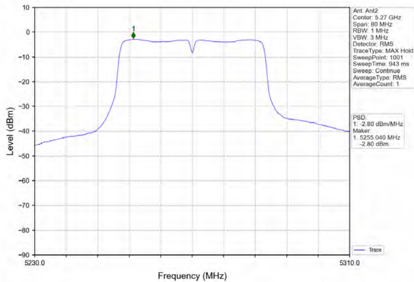
802.11n(HT40)_LCH_5270MHz_MIMO_NTNV
