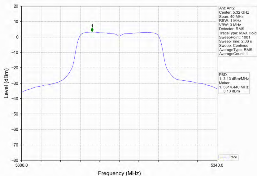
802.11a_HCH_5320MHz_Ant2_NTNV
