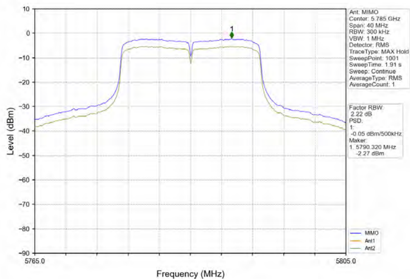
802.11n(HT20)_MCH_5785MHz_MIMO_NTNV
