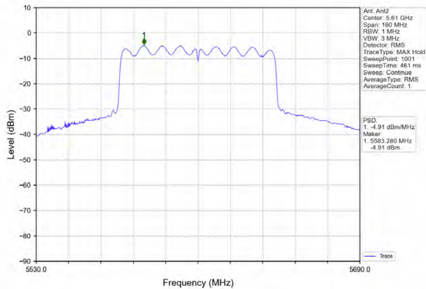
802.11ac(VHT80)_HCH_5610MHz_MIMO_NTNV
