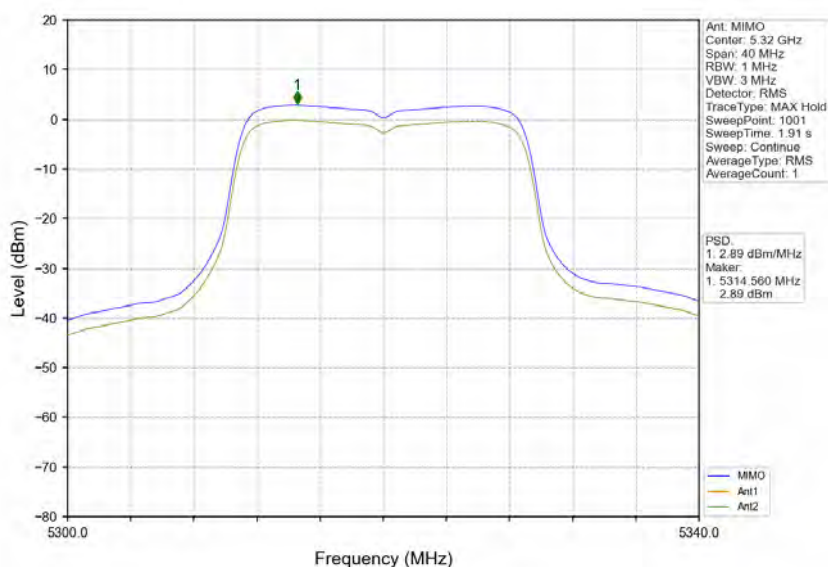
802.11n(HT20)_HCH_5320MHz_MIMO_NTNV
