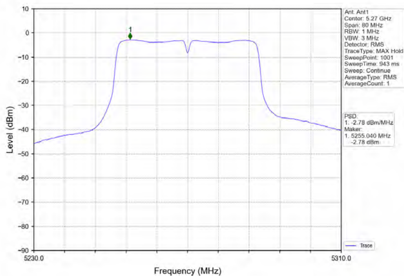
802.11n(HT40)_LCH_5270MHz_Ant1_NTNV
