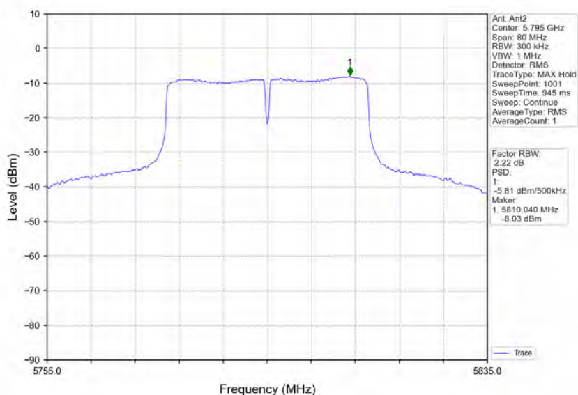
802.11n(HT40)_HCH_5795MHz_Ant2_NTNV
