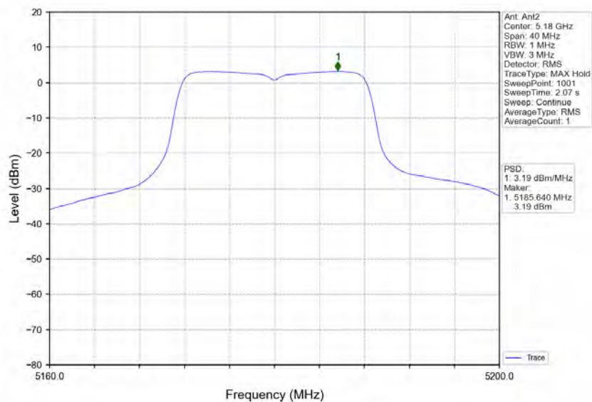
802.11a_LCH_5180MHz_Ant2_NTNV
