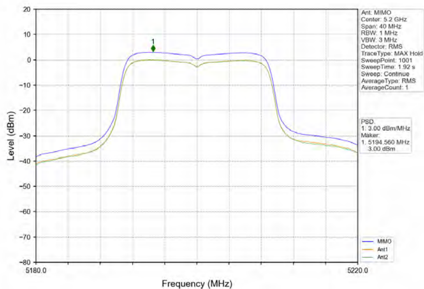
802.11n(HT20)_MCH_5200MHz_MIMO_NTNV
