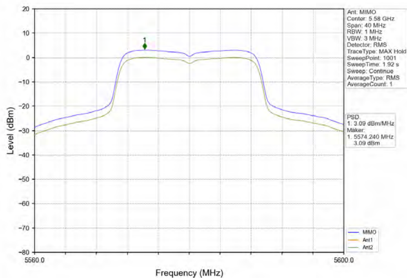
802.11n(HT20)_MCH_5580MHz_MIMO_NTNV
