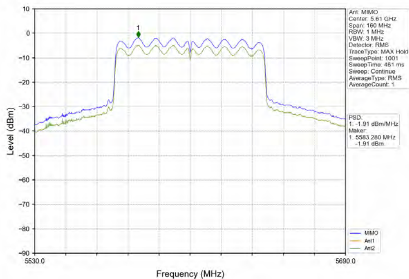
802.11ac(VHT80)_HCH_5610MHz_MIMO_NTNV
