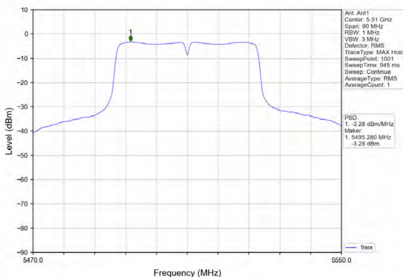
802.11n(HT40)_LCH_5510MHz_Ant1_NTNV
