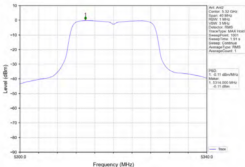
802.11n(HT20)_HCH_5320MHz_MIMO_NTNV
