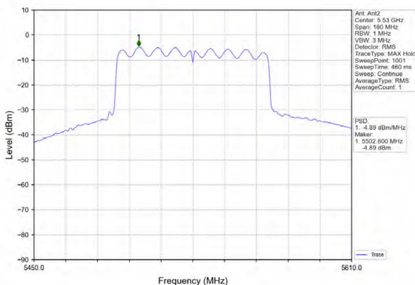
802.11ac(VHT80)_LCH_5530MHz_Ant2_NTNV
