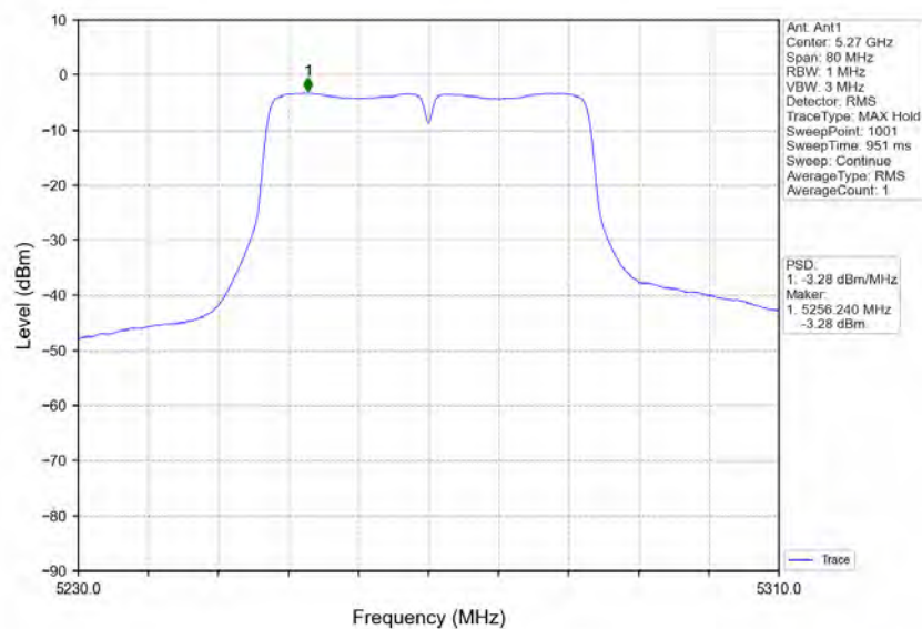
802.11ac(VHT40)_LCH_5270MHz_Ant1_NTNV
