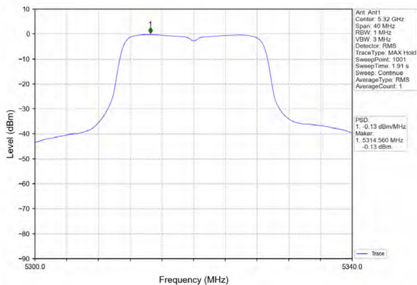
802.11n(HT20)_HCH_5320MHz_Ant1_NTNV
