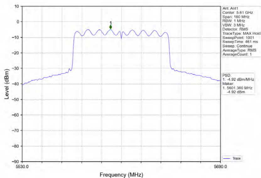
802.11ac(VHT80)_HCH_5610MHz_Ant1_NTNV
