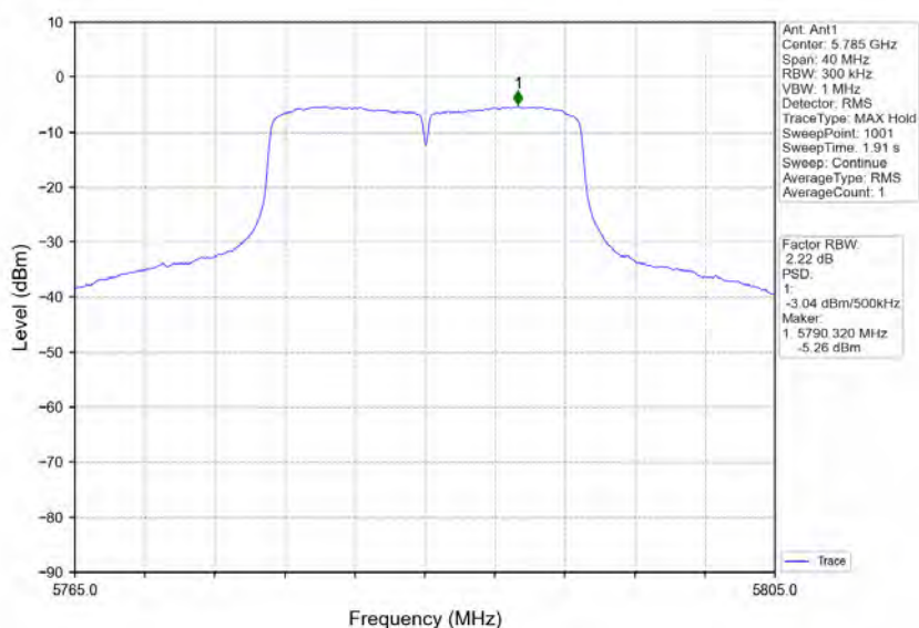
802.11n(HT20)_MCH_5785MHz_Ant1_NTNV
