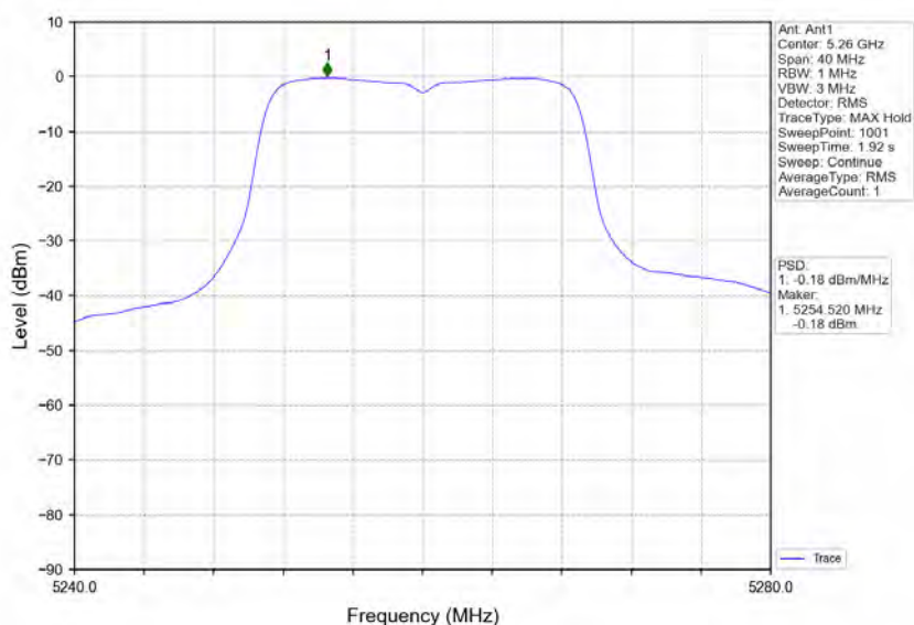
802.11n(HT20)_LCH_5260MHz_Ant1_NTNV
