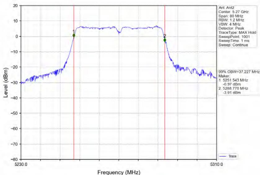
802.11n(HT40)_LCH_5270MHz_Ant2_NTNV
