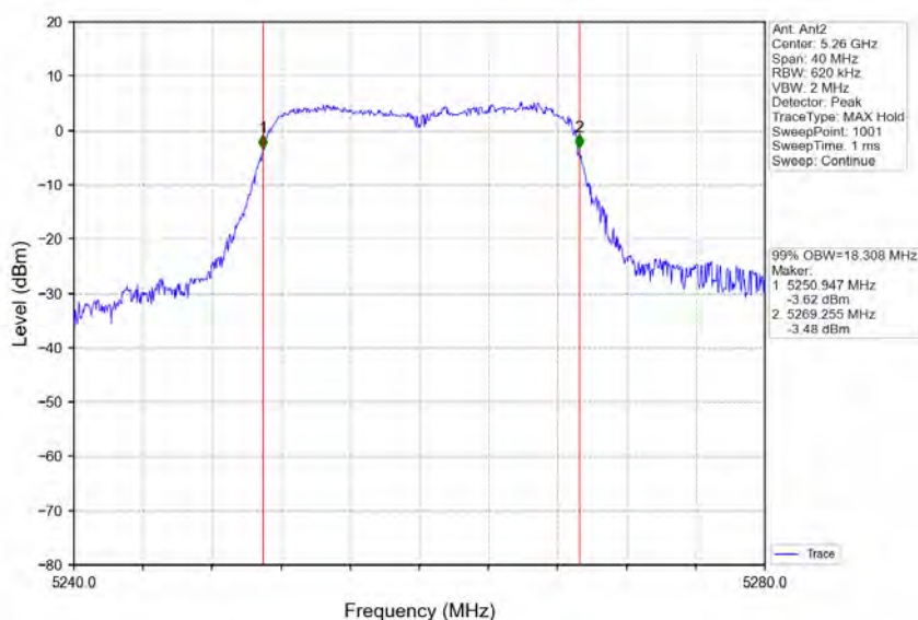
802.11n(HT20)_LCH_5260MHz_Ant2_NTNV
