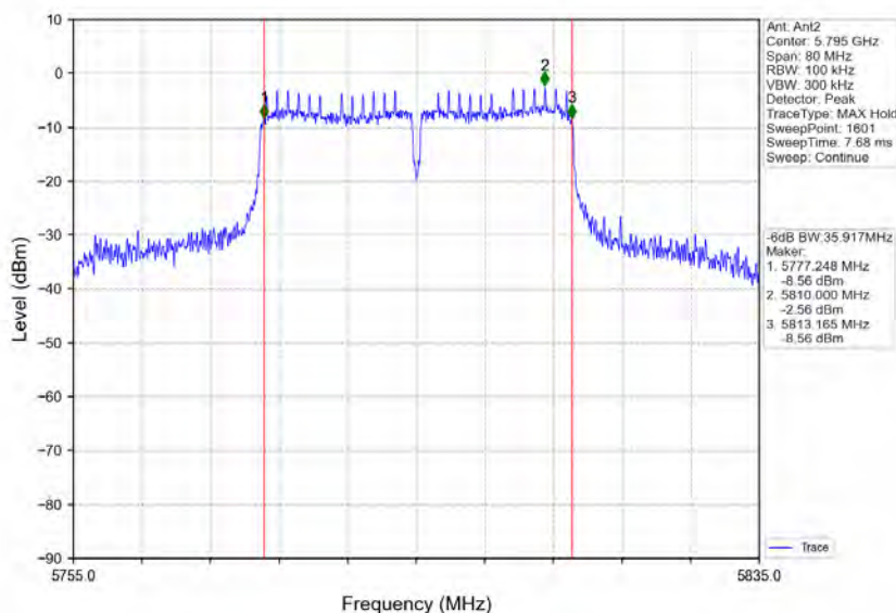
802.11n(HT40)_HCH_5795MHz_Ant2_NTNV
