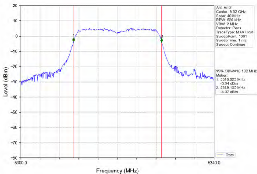
802.11n(HT20)_HCH_5320MHz_Ant2_NTNV
