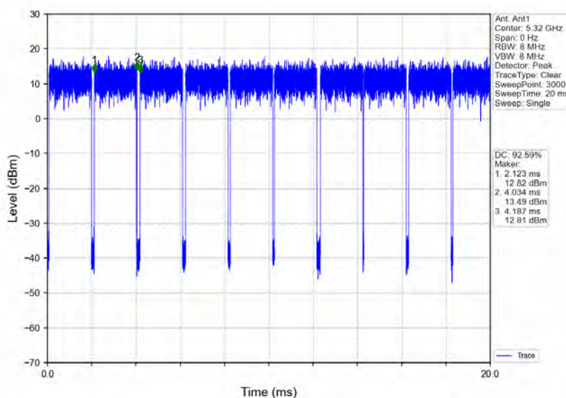
802.11n(HT20)_HCH_5320MHz_Ant1_NTNV
