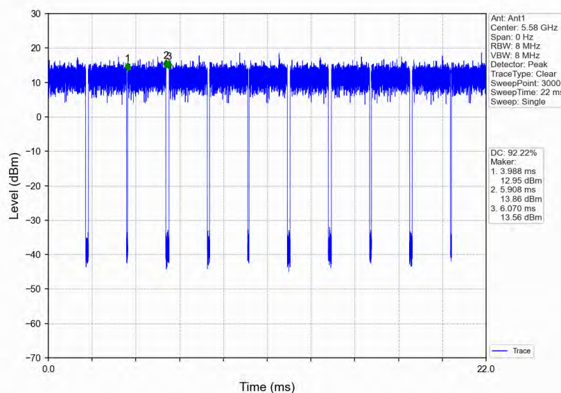
802.11n(HT20)_MCH_5580MHz_Ant1_NTNV
