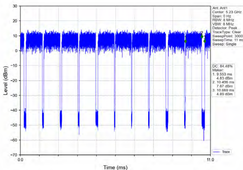
802.11n(HT40)_HCH_5230MHz_Ant1_NTNV
