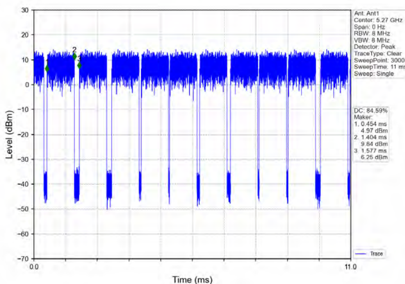
802.11ac(VHT40)_LCH_5270MHz_Ant1_NTNV
