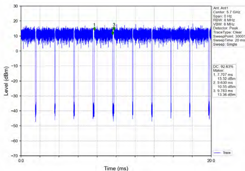
802.11ac(VHT20)_HCH_5700MHz_Ant1_NTNV
