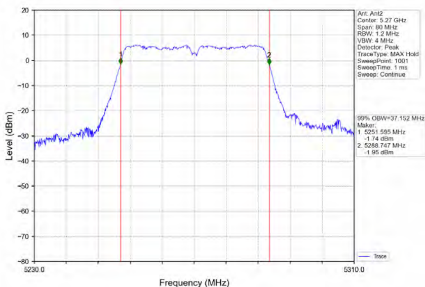
802.11ac(VHT40)_LCH_5270MHz_Ant2_NTNV
