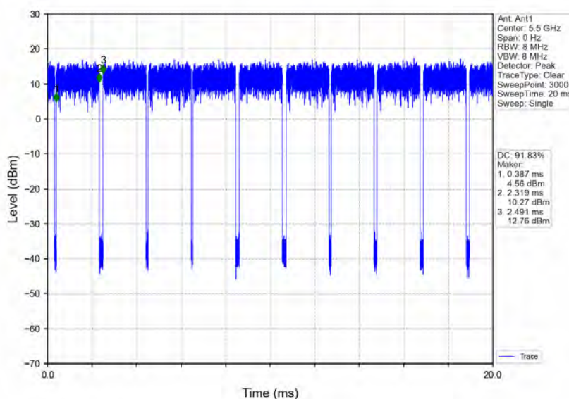
802.11ac(VHT20)_LCH_5500MHz_Ant1_NTNV
