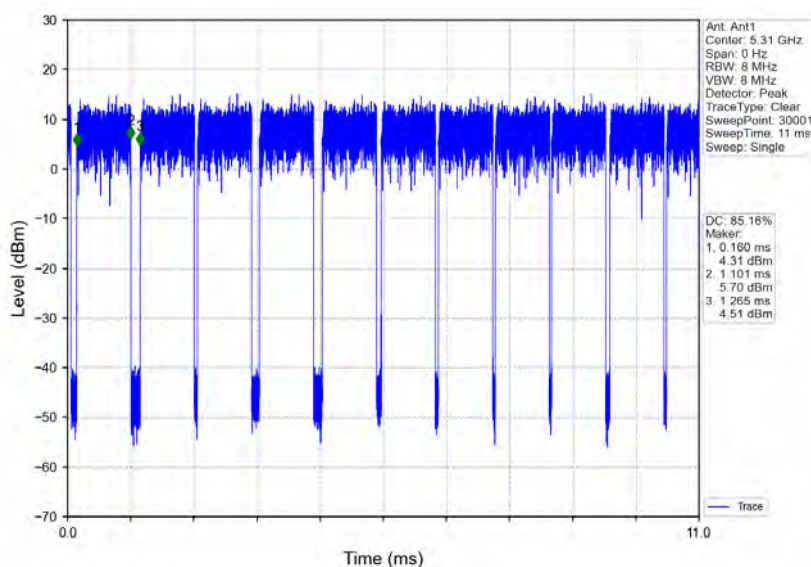
802.11n(HT40)_HCH_5310MHz_Ant1_NTNV
