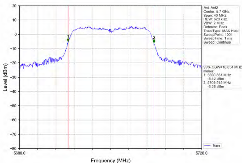
802.11n(HT20)_HCH_5700MHz_Ant2_NTNV
