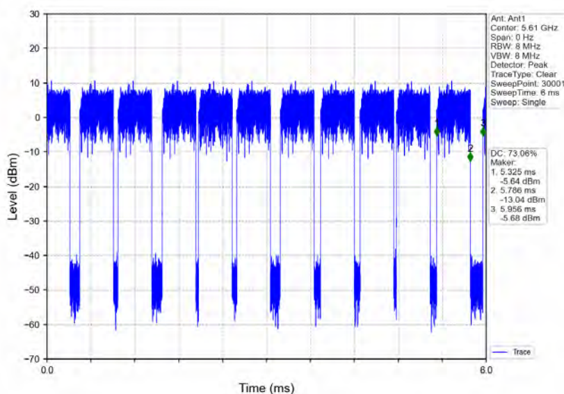
802.11ac(VHT80)_HCH_5610MHz_Ant1_NTNV
