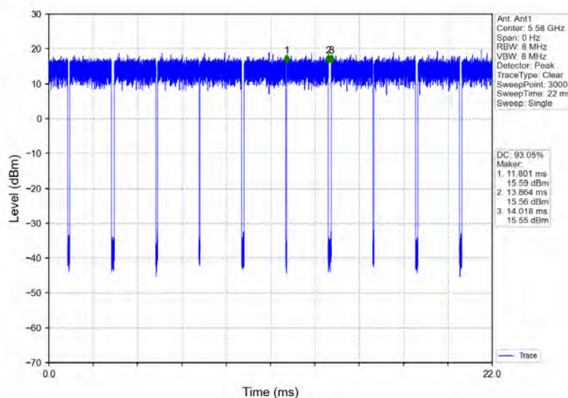
802.11a_MCH_5580MHz_Ant1_NTNV
