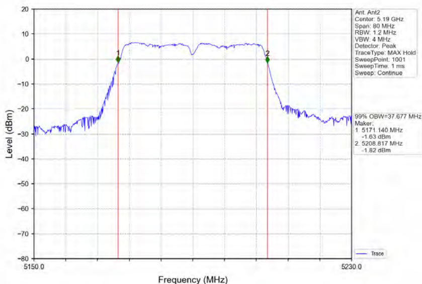
802.11n(HT40)_LCH_5190MHz_Ant2_NTNV
