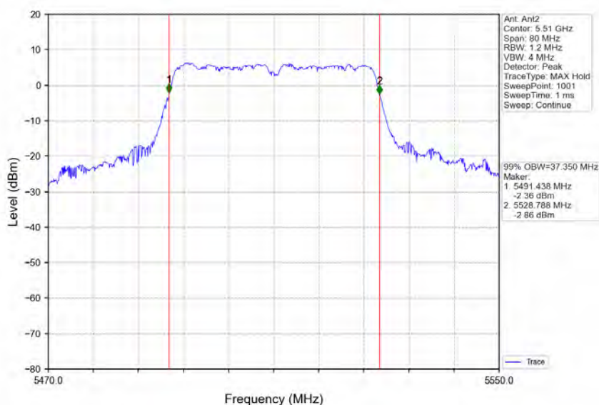
802.11n(HT40)_LCH_5510MHz_Ant2_NTNV
