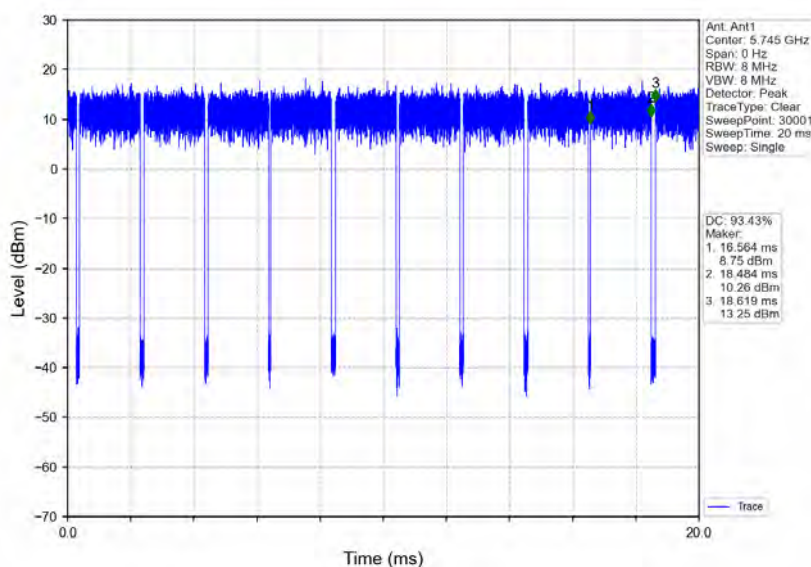
802.11n(HT20)_LCH_5745MHz_Ant1_NTNV
