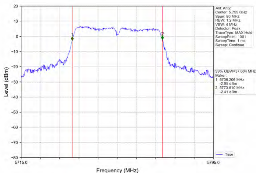
802.11n(HT40)_LCH_5755MHz_Ant2_NTNV
