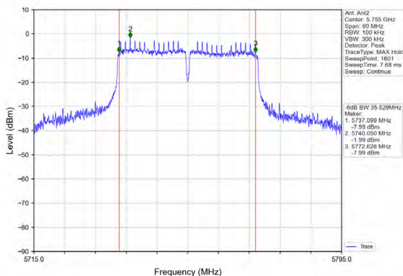
802.11n(HT40)_LCH_5755MHz_Ant2_NTNV
