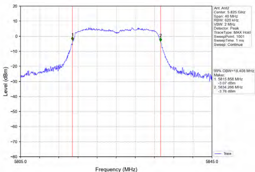
802.11n(HT20)_HCH_5825MHz_Ant2_NTNV
