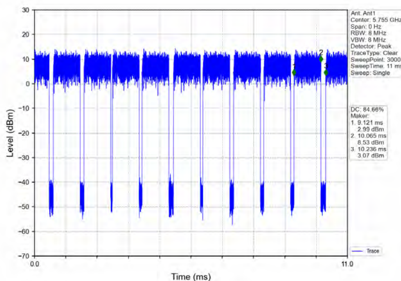
802.11n(HT40)_LCH_5755MHz_Ant1_NTNV
