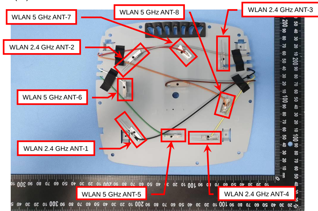
EUT Photo (14)
