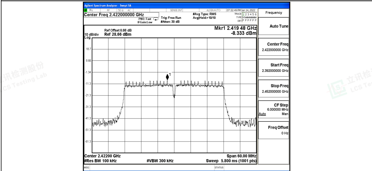
11N40SISO_Ant_2422_30~100
