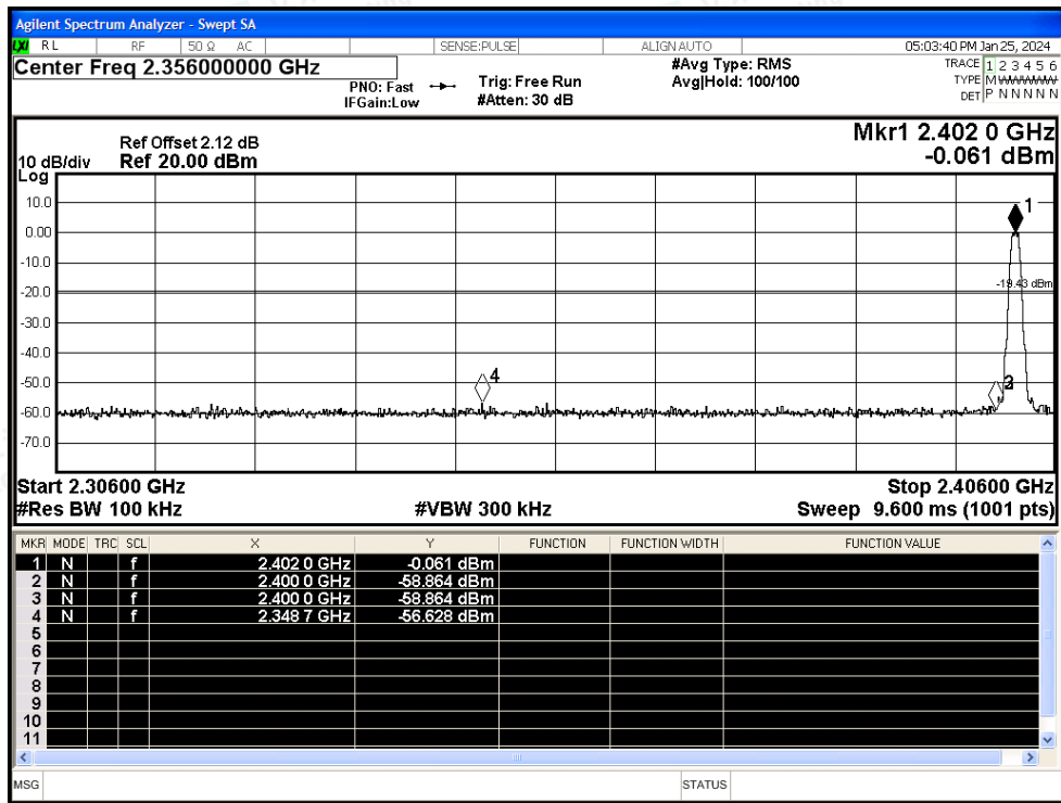
Band Edge NVNT BLE 1M 2402MHz Ant Emission
