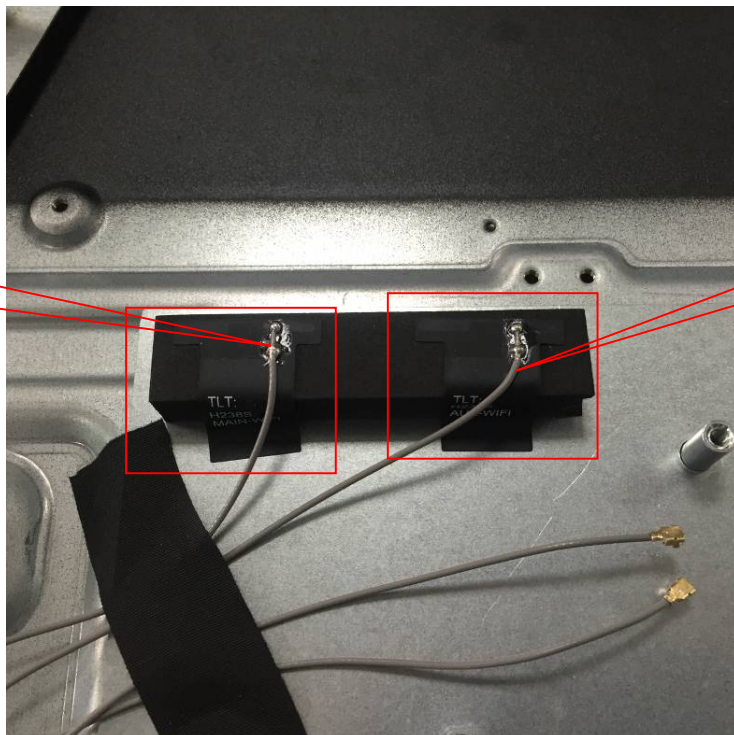
FPC Antennas
