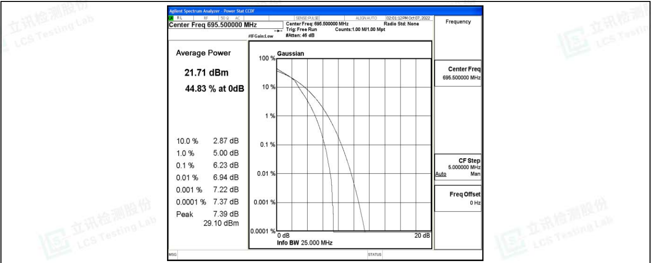
Band71-10MHz-QPSK-133172-50RB#0
