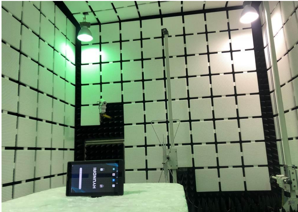
Fig. 1 (Below 1GHz)
