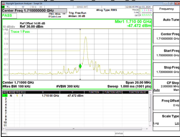
Band Edge_Band4_10MHz_QPSK_RB1_5_CH20350
