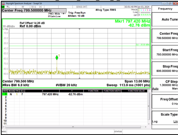
Band13_10MHz_QPSK_RB1_5_CH23230
