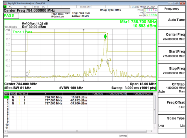
Band Edge_Band13_5MHz_QPSK_RB1_5_CH23255
