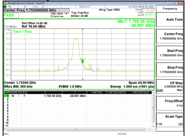
Band Edge_Band4_20MHz_QPSK_RB6_0_CH20300
