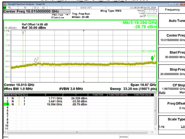
Band4_20MHz_QPSK_RB1_0_CH20175
