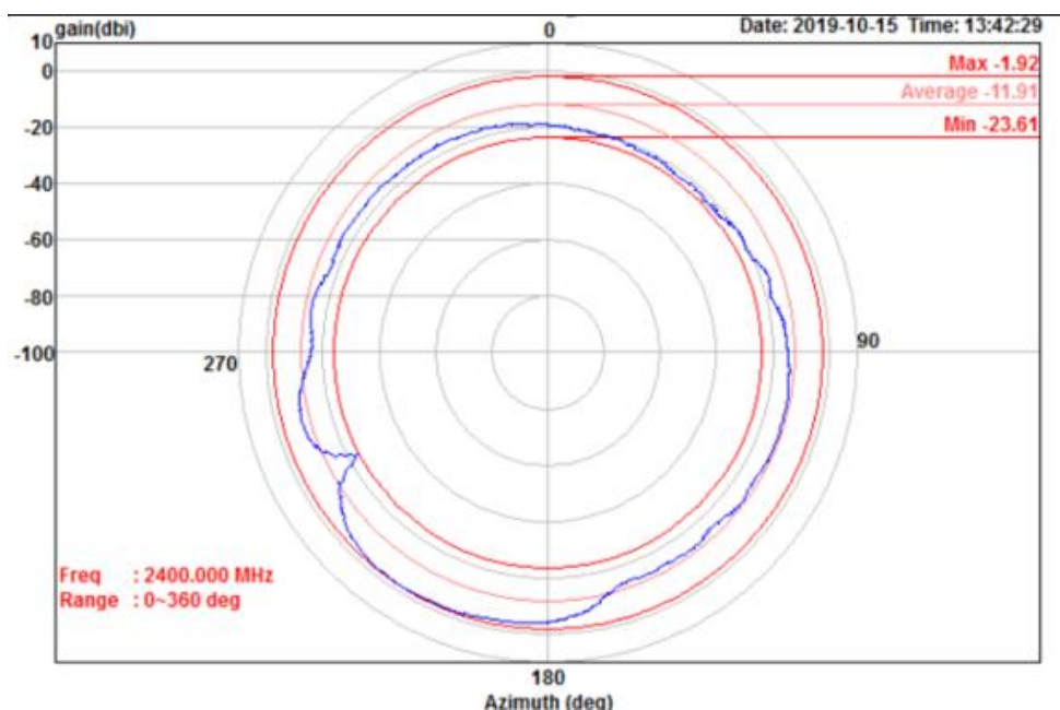
Figure1. 2.4G Antenna 2400MHz
