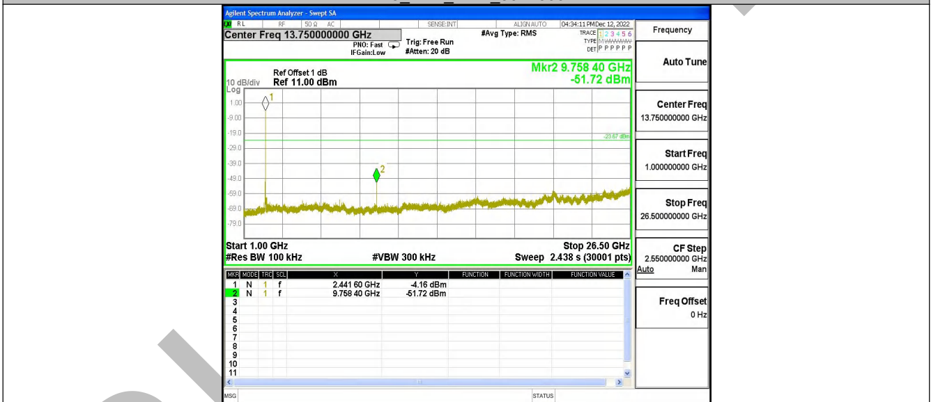
DH5 Ant1 2441 1000~26500
