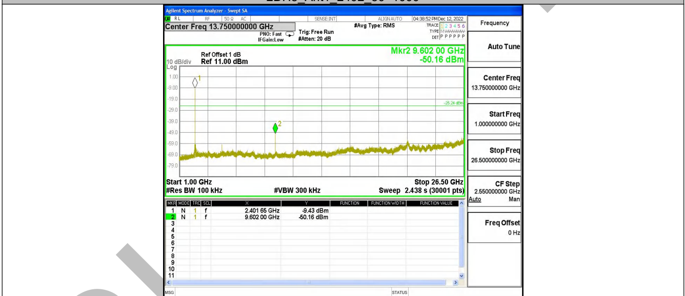
2DH5_Ant1_2402_1000~26500
