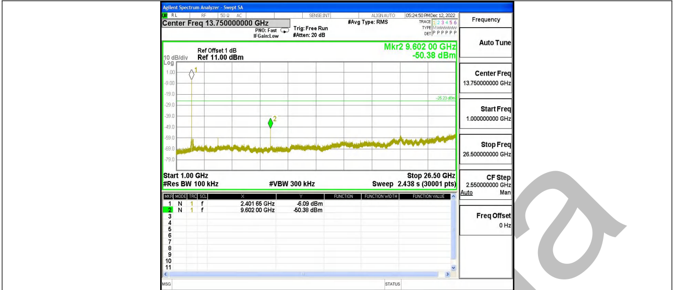
DH5_Ant1_2402_1000~26500
