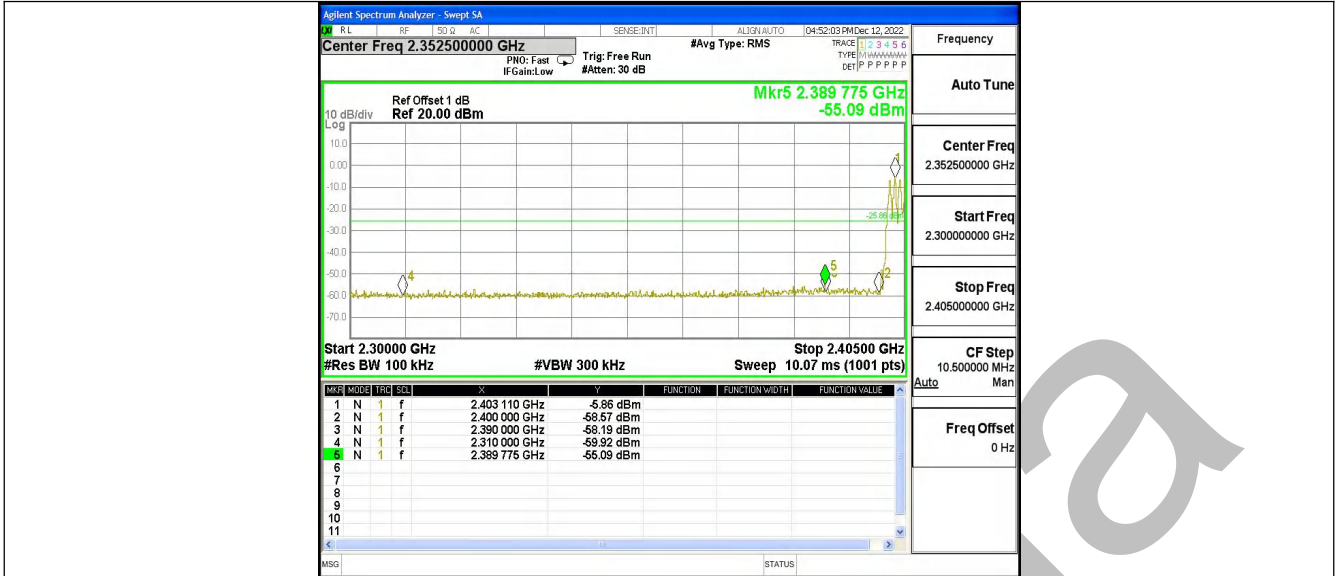
DH5_Ant1_Low_Hop_2402
