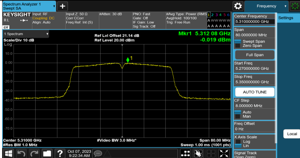
11N40MIMO Ant2 5310
