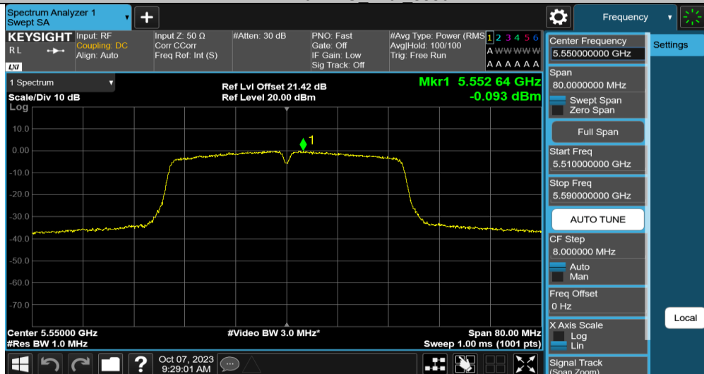
11N40MIMO Ant2 5550
