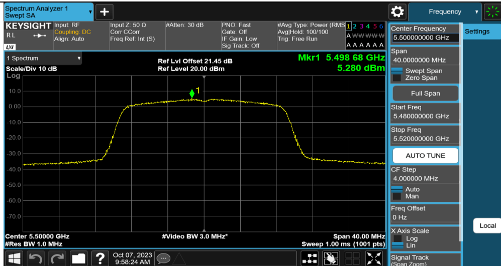
11AC20MIMO_Ant2_5500
