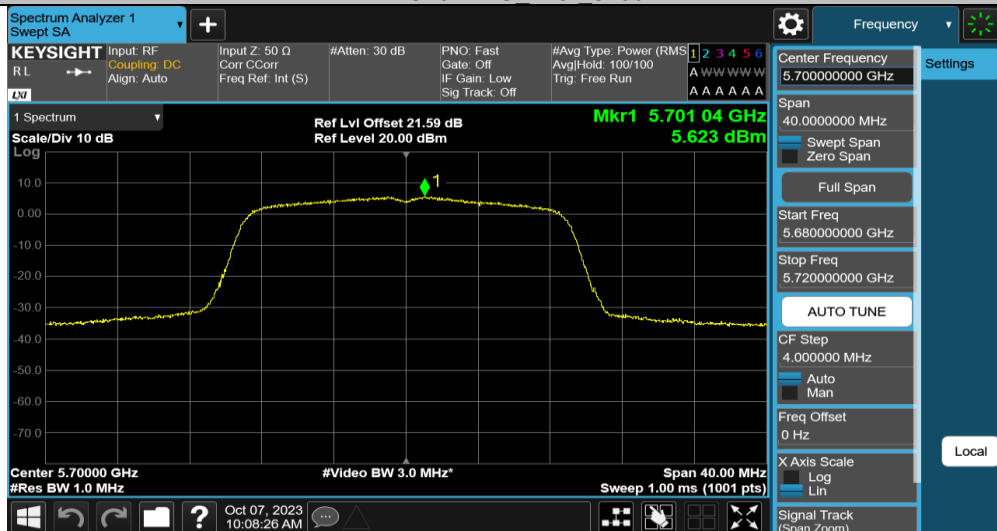
11AC20MIMO_Ant2_5700
