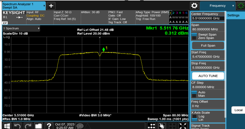
11N40MIMO Ant2 5510
