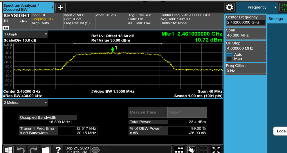
11G-CDD Ant2 2462
