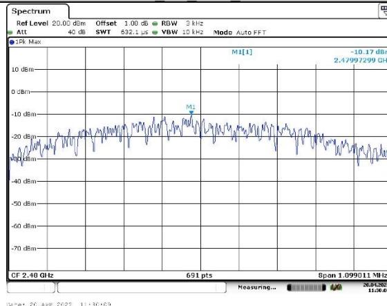
BLE 1M Ant1 2480
