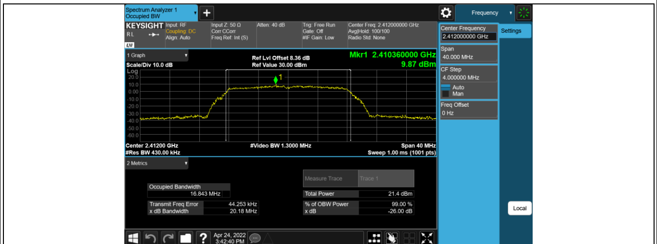
11G-CDD Ant1 2437
