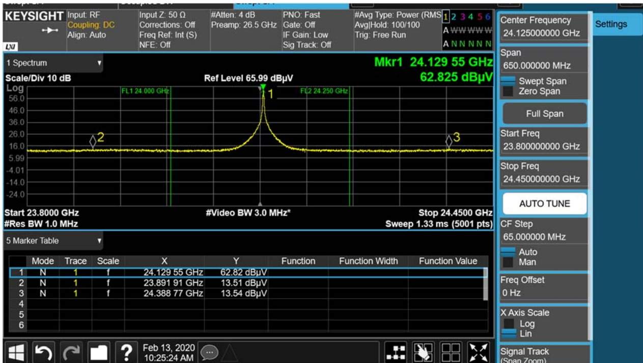
Band Edge Plot(average, x-V)
