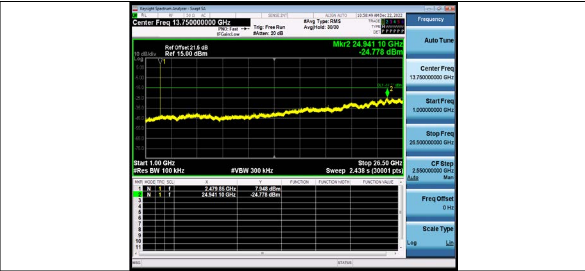
BLE_500K_Ant1_2402_0~Reference
