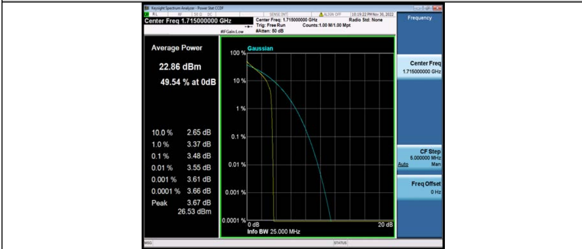
Band66-10MHz-QPSK-132022-50RB#0
