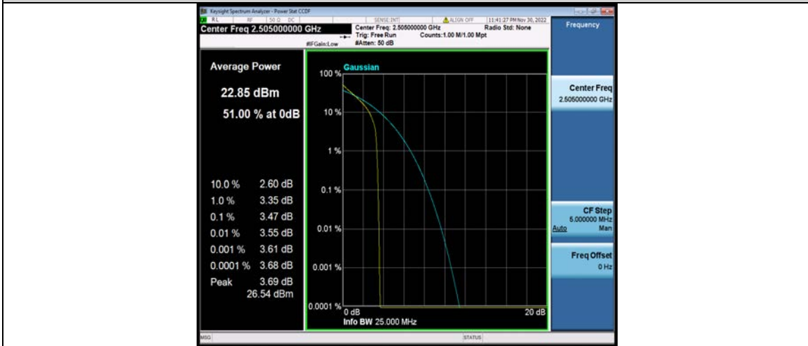
Band7-10MHz-QPSK-20800-50RB#0
