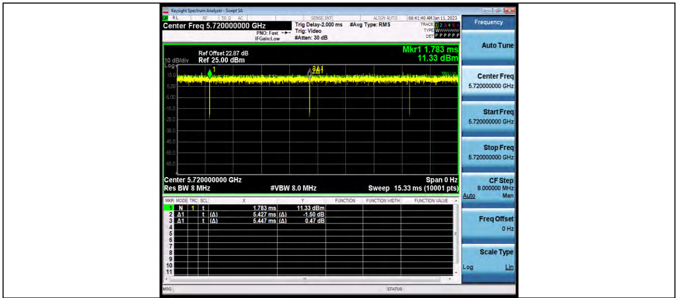
11AC20MIMO_Ant2_5720
