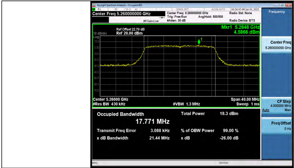
11N20MIMO_Ant2_5260
