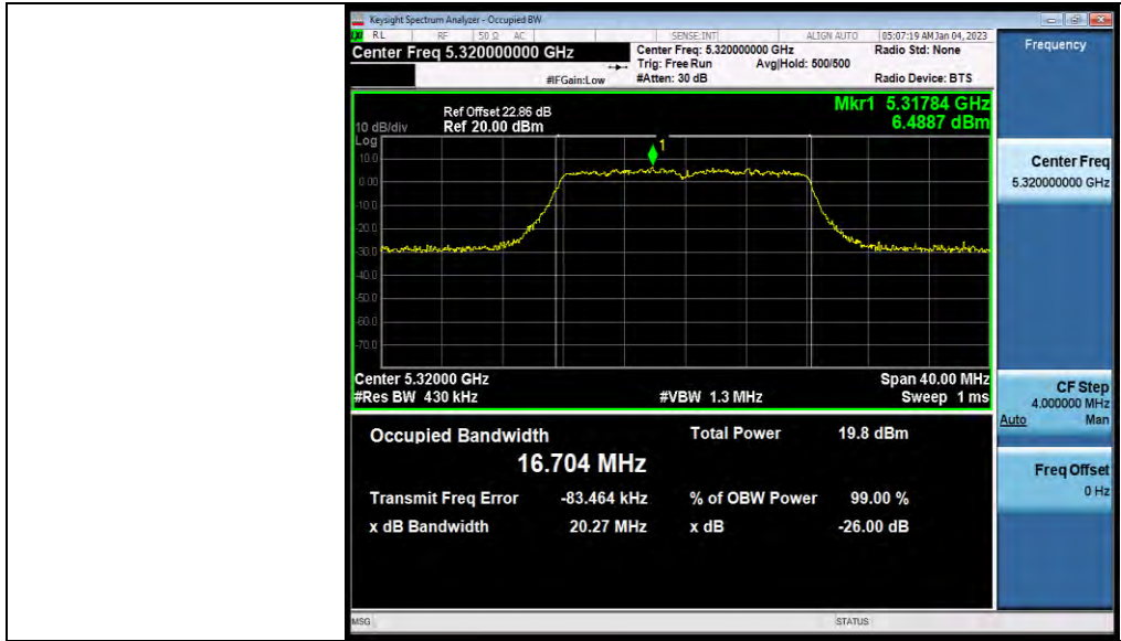
11A-CDD_Ant2_5320
