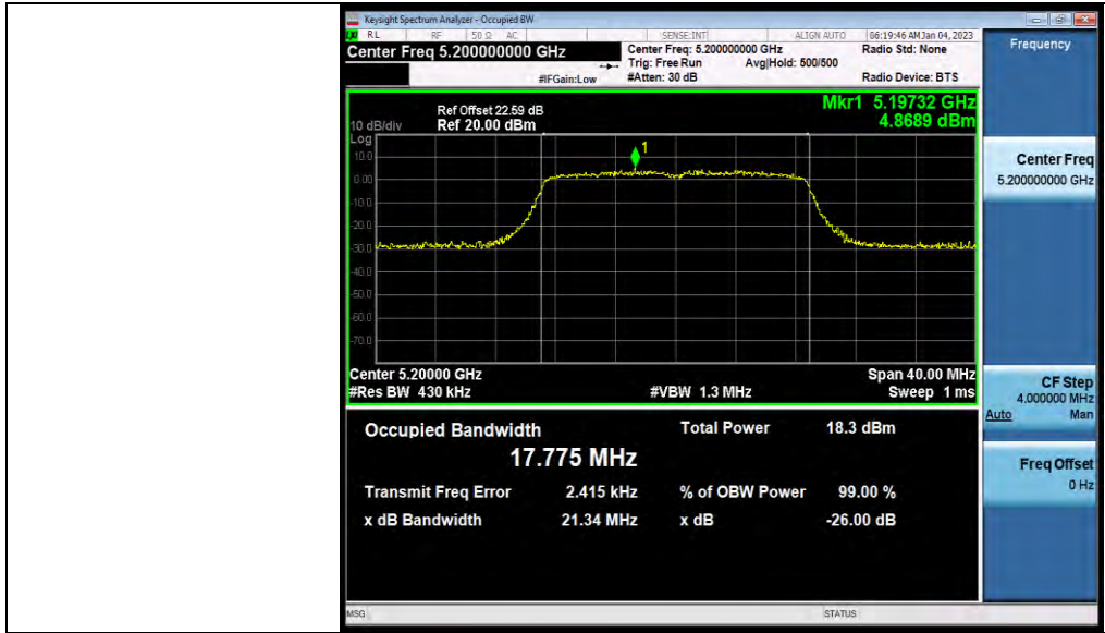
11N20MIMO_Ant2_5200
