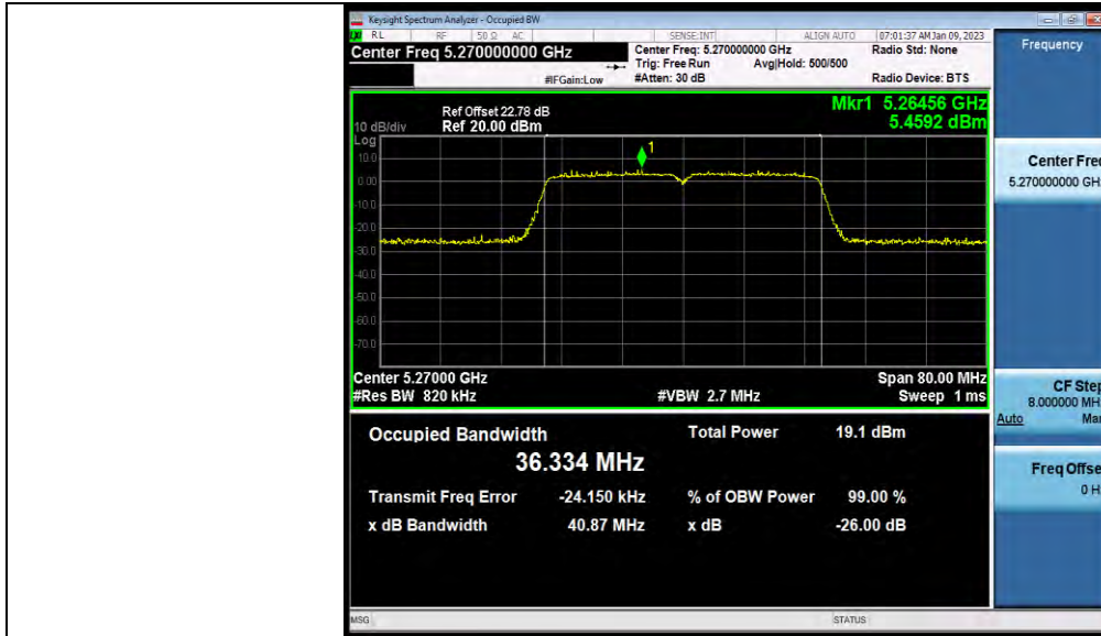
11N40MIMO_Ant2_5270
