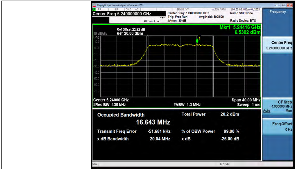
11A-CDD_Ant2_5240
