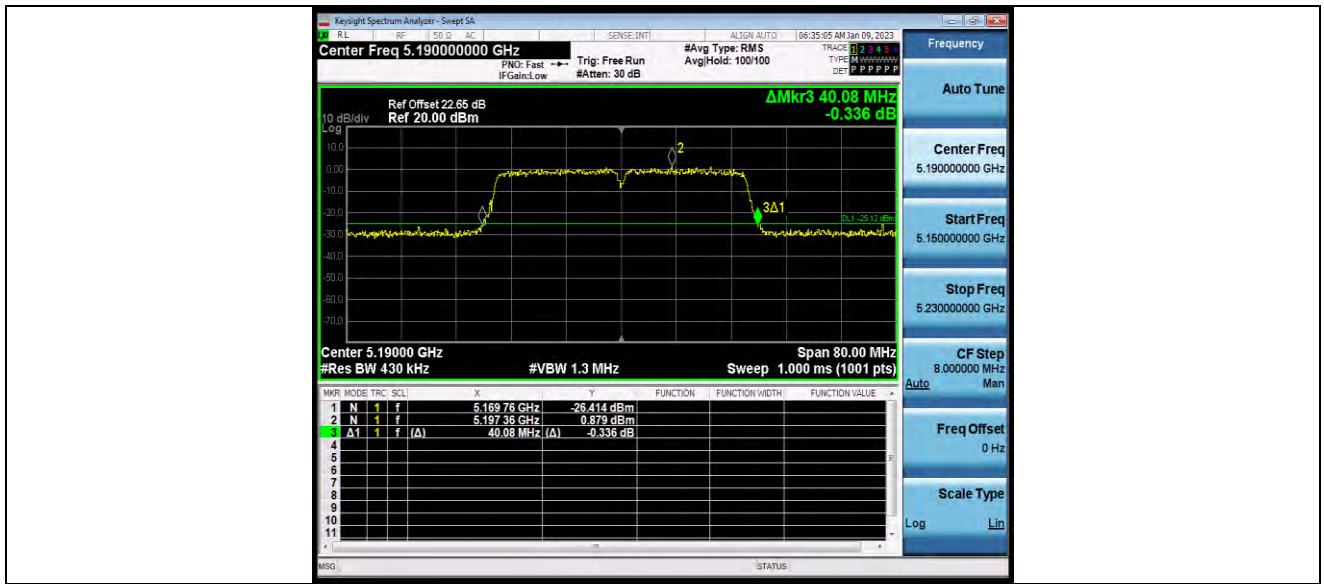
11N40MIMO_Ant2_5190
