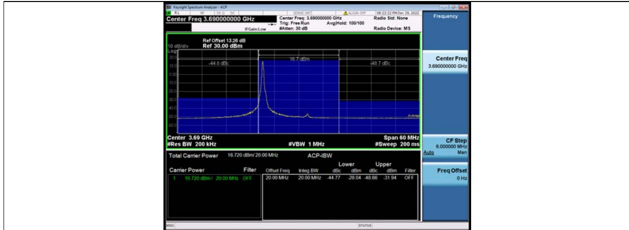
Band48-20MHz-QPSK-56640-1RB#99
