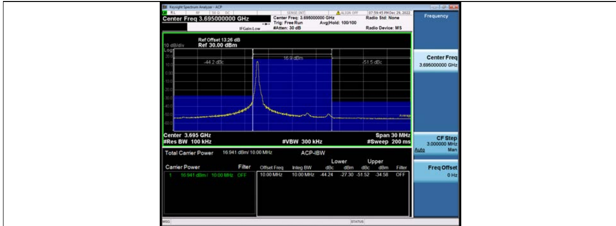
Band48-10MHz-QPSK-56690-50RB#0
