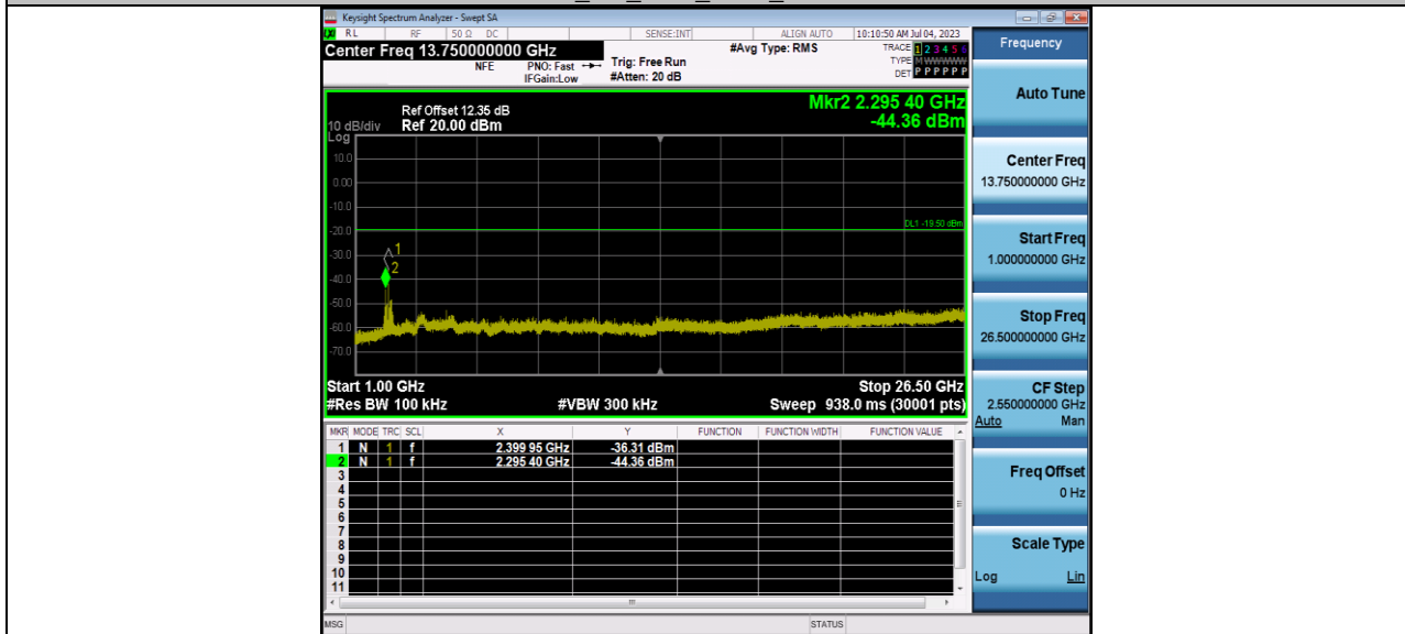
BLE_2M_Ant1_2402_1000~26500
