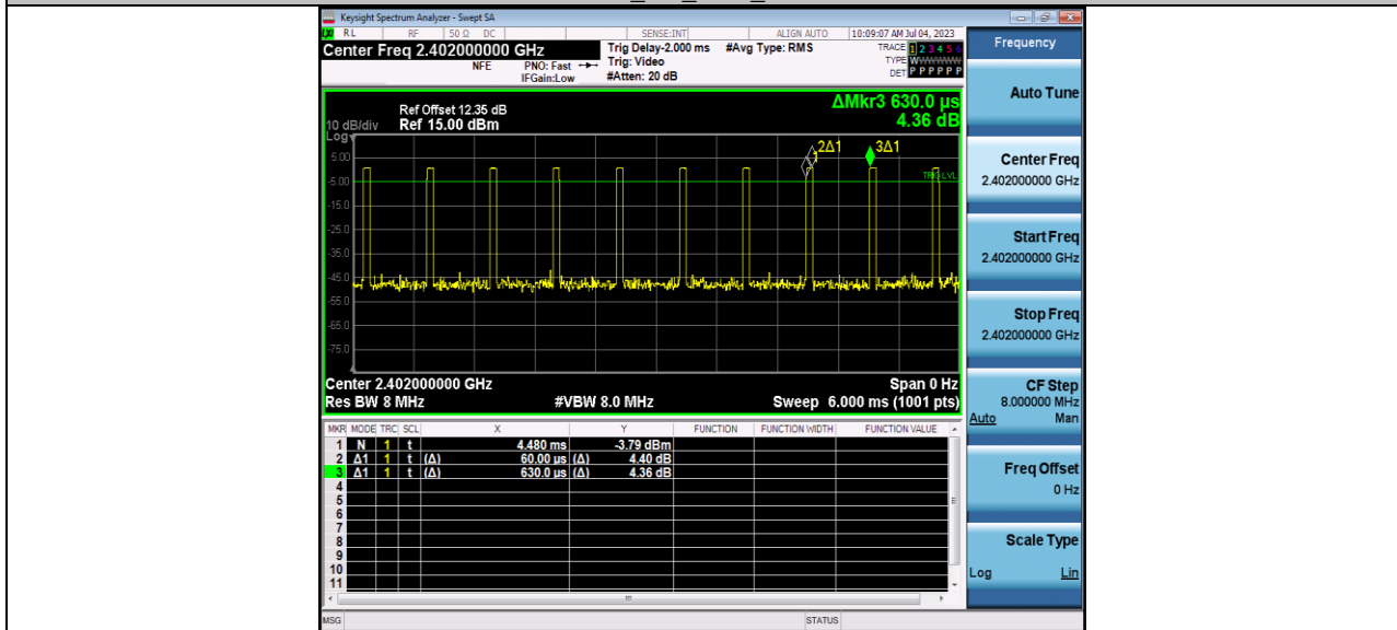
BLE_2M_Ant1_2402
