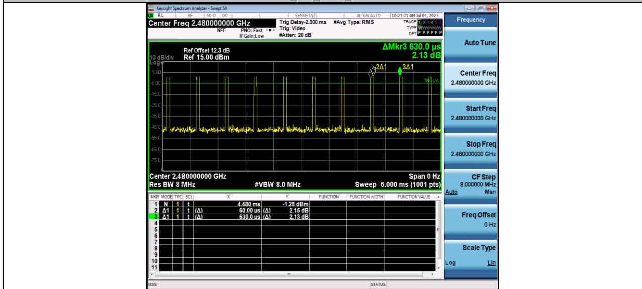
BLE_2M_Ant1_2480
