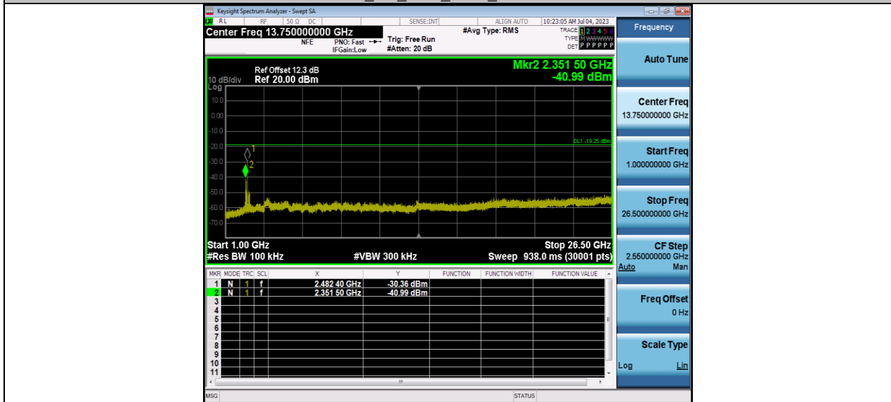
BLE_2M_Ant1_2480_1000~26500
