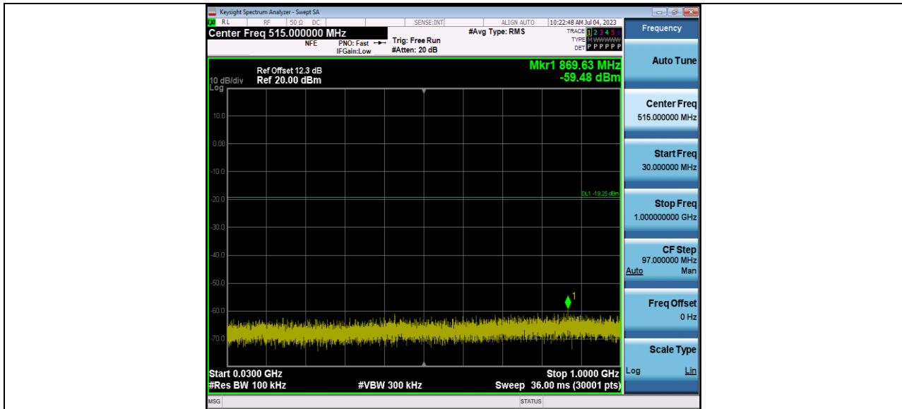
BLE_2M_Ant1_2480_30~1000
