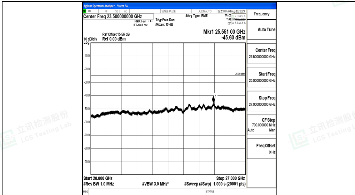
Band7_20MHz_QPSK_20850_1RB#0_20000~27000_20000~27000
