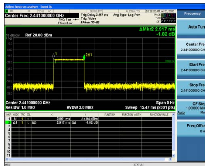
2-DH5
