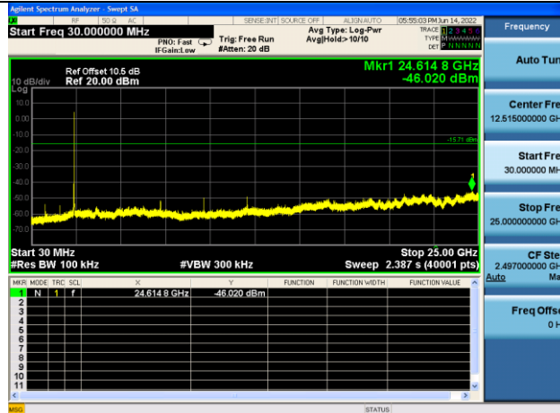
802.11b,2437MHz,Ant0,Plot 2,30MHz~2 5000MHz
