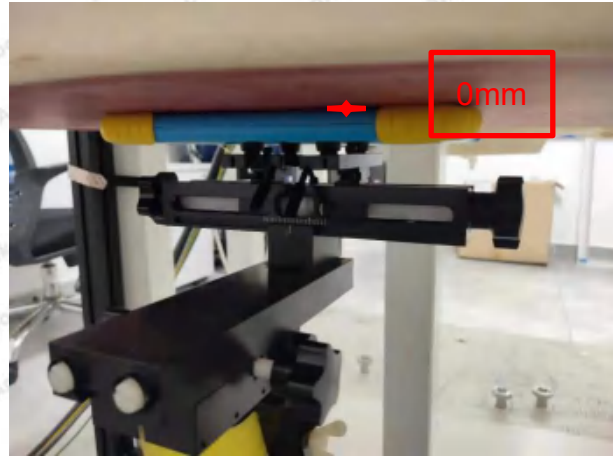
Body Front(0mm)
