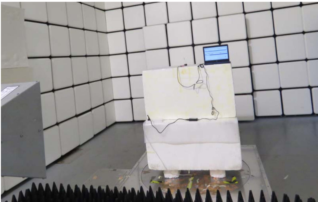
1GHz-18GHz
