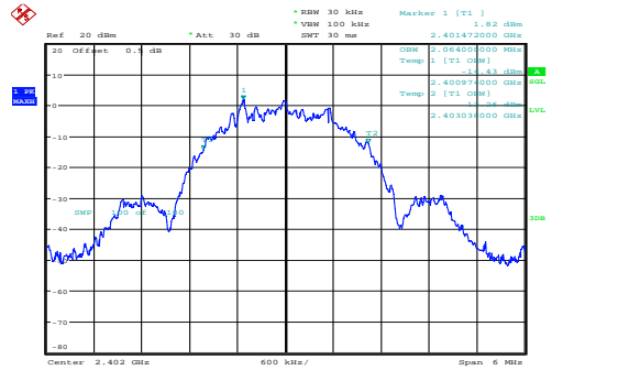
Low 2.064MHz
