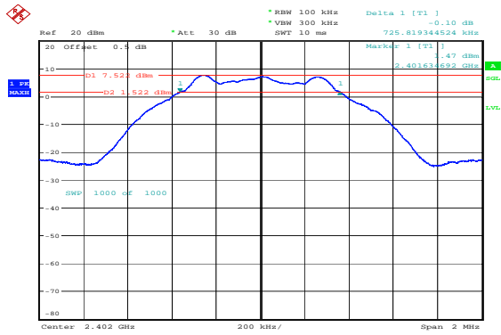
Low 0.726MHz
