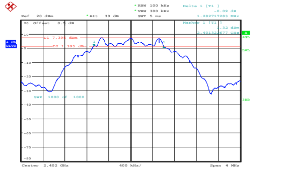
Low 1.283MHz
