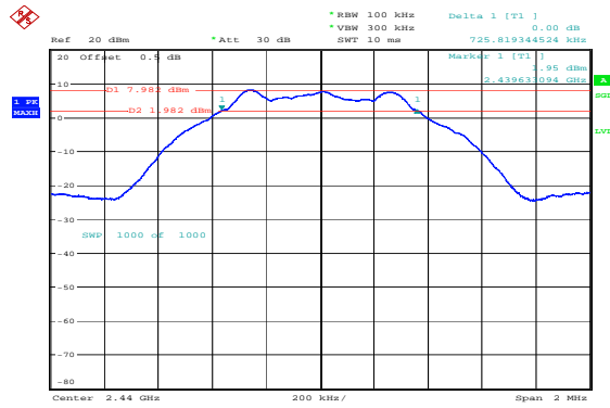
Middle 0.726MHz
