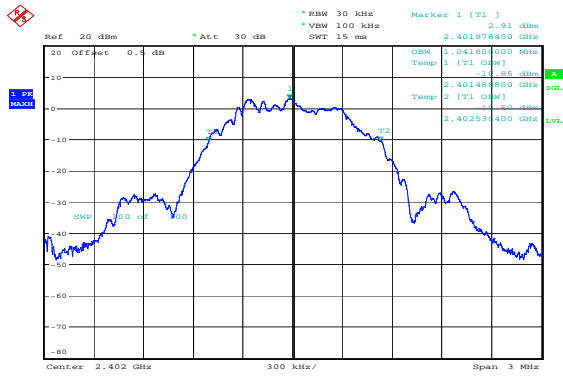
Low 1.042MHz
