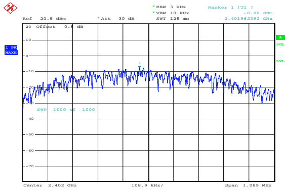
Low -8.08dBm/3kHz
