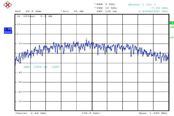
Middle -7.54dBm/3kHz
