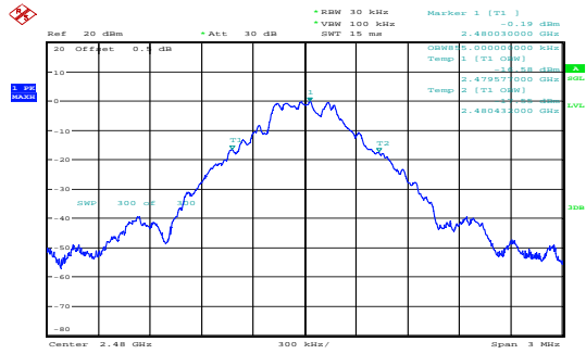
GFSK_High 0.855MHz
