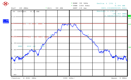
GFSK_Middle 0.965MHz
