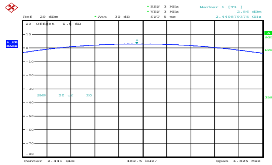
GFSK_Middle 2.86dBm
