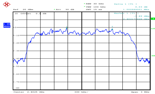
\pi/4 -DQPSK_Low 1.001MHz
