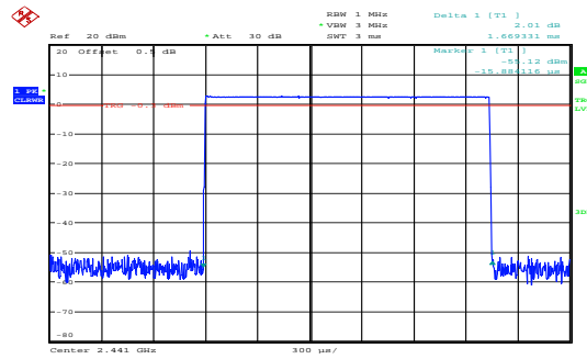
GFSK_Hopping_DH3 1.669ms
