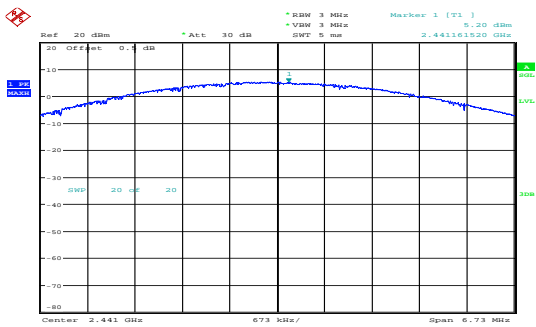
\pi/4 -DQPSK_Middle 5.20dBm
