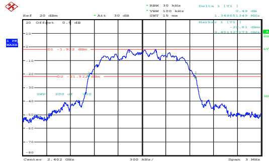
\pi/4 -DQPSK_Low 1.349MHz
