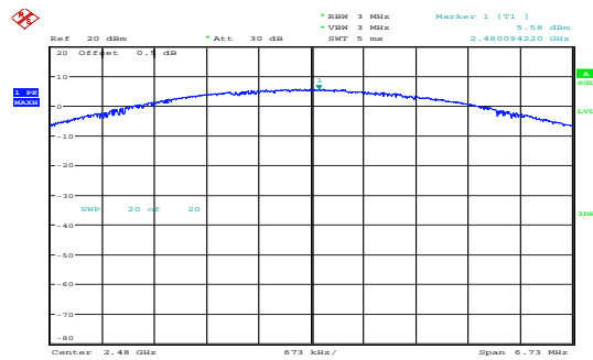
\pi/4 -DQPSK_High 5.58dBm
