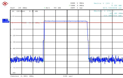
GFSK_Hopping_DH1 0.404ms
