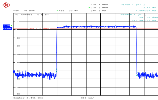
\pi/4 -DQPSK_Hopping_2DH3 1.666ms
