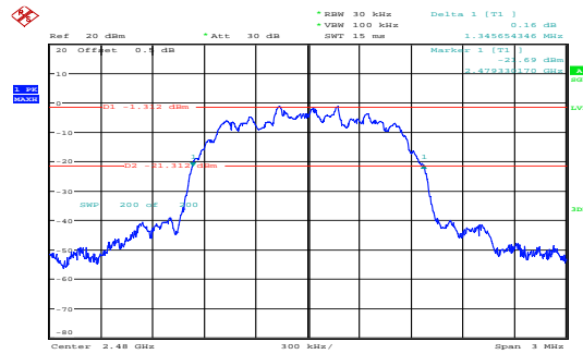
\pi/4 -DQPSK_High 1.346MHz
