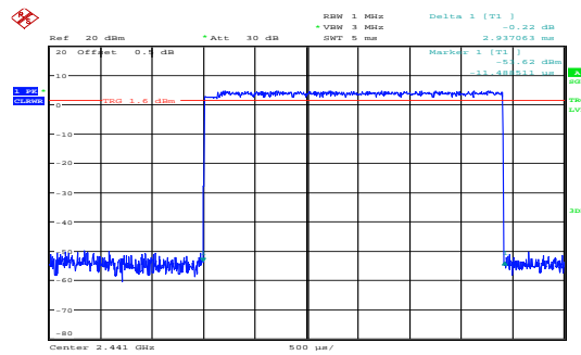
\pi/4 -DQPSK_Hopping_2DH5 2.937ms
