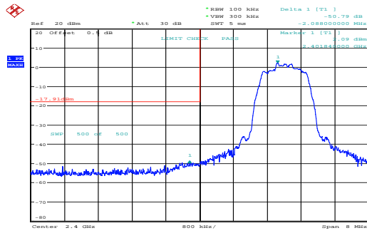
\pi/4 -DQPSK_Low 50.79dB
