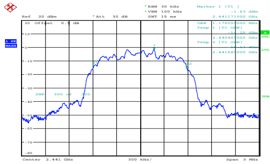
\pi/4 -DQPSK_Middle 1.176MHz
