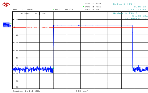
GFSK_Hopping_DH5 2.937ms
