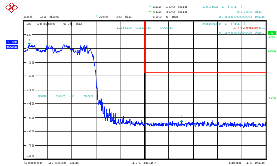
\pi/4 -DQPSK_Hopping_Upper 54.83dB
