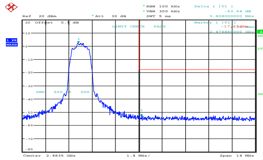
\pi/4 -DQPSK_High 53.94dB
