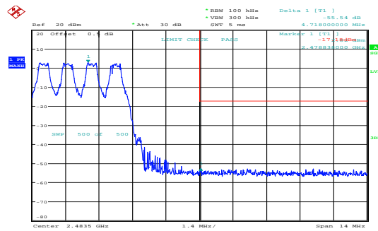
GFSK_Hopping_Upper 55.54dB
