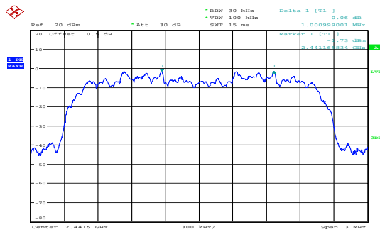
\pi/4 -DQPSK_Middle 1.001MHz
