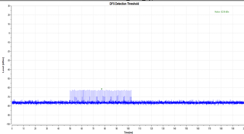
11AX160MIMO_5250_Type1
