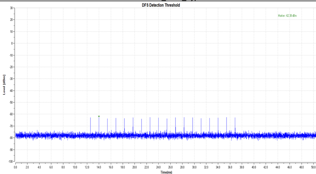
11AX20MIMO_5580_Type1
