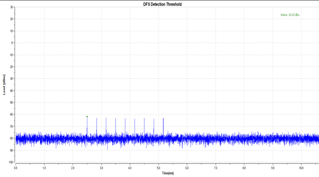
11AX160MIMO_5250_Type0
