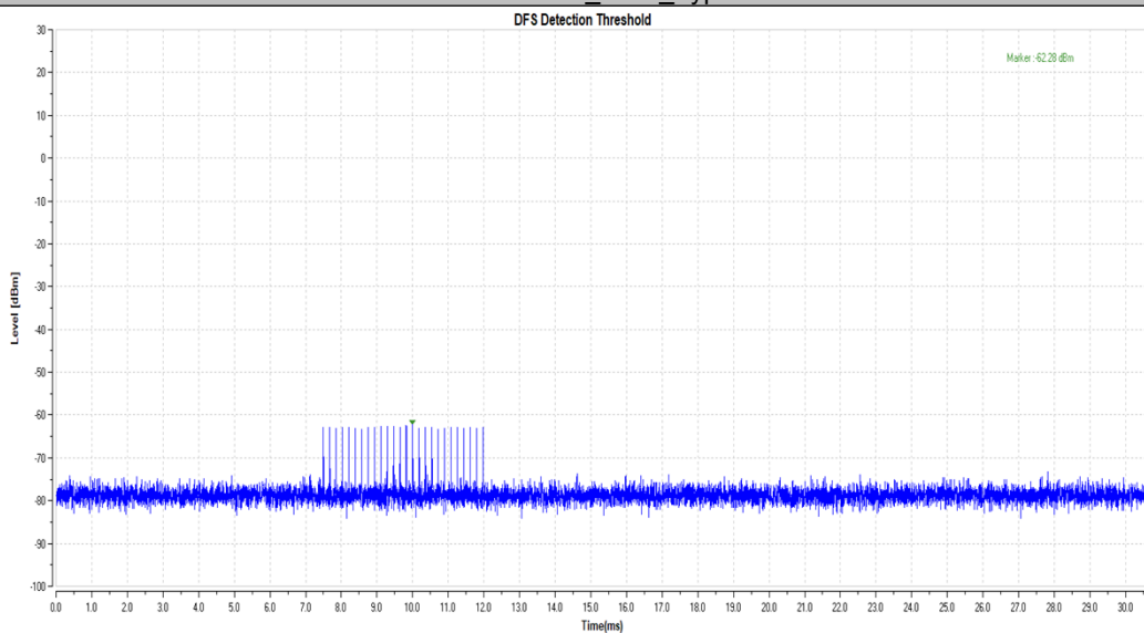
11AX20MIMO_5580_Type2
