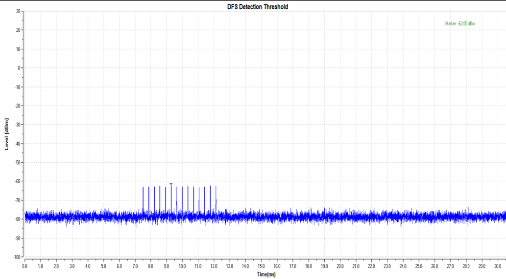
11AX20MIMO_5580_Type5
