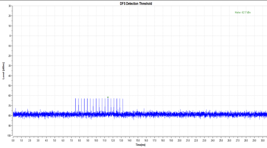
11AX20MIMO_5580_Type4
