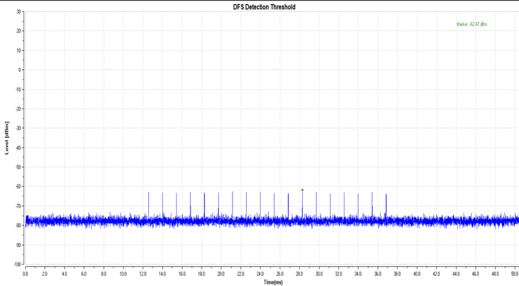
11AX160MIMO_5250_Type1
