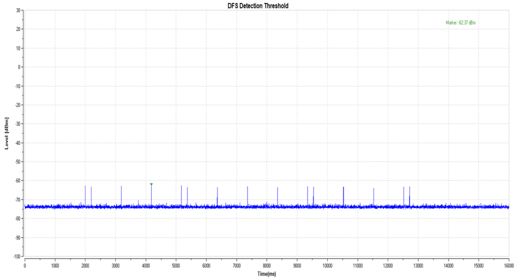
11AX160MIMO_5250_Type6
