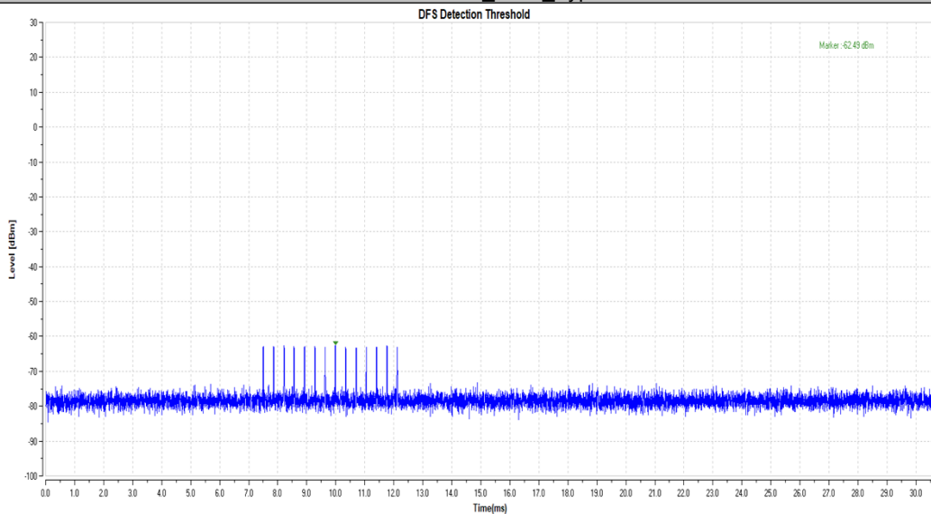
11AX160MIMO_5250_Type4
