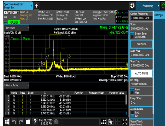
SCC_20M_3569.9MHz_Q16_1RB_CSEpart96
