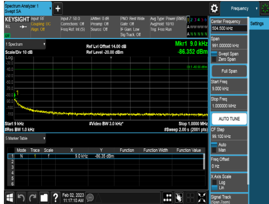
SCC_20M_3630MHz_Q16_FULLLRB_CSE1
