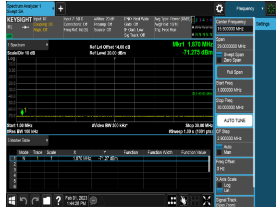
SCC_20M_3630MHz_Q16_FULLLRB_CSE2
