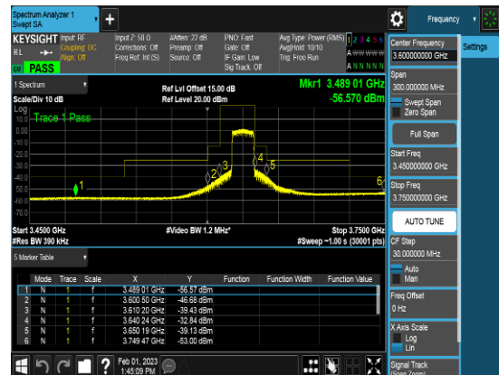
SCC_20M_3630MHz_Q16_FULLLRB_CSEpart96
