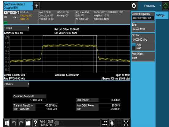
SCC_20M_3690MHz_QPSK_FULLLRB_OBW
