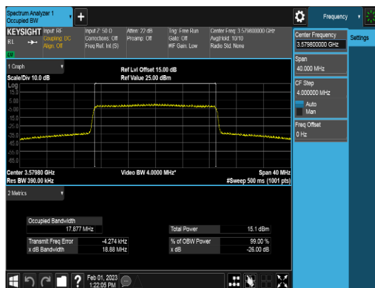
SCC_20M_3579.8MHz_Q64_FULLLRB_OBW
