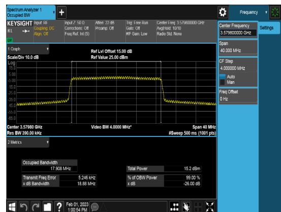
SCC_20M_3579.8MHz_QPSK_FULLLRB_OBW
