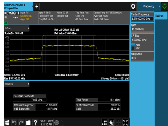
SCC_20M_3579.8MHz_QPSK_FULLLRB_OBW
