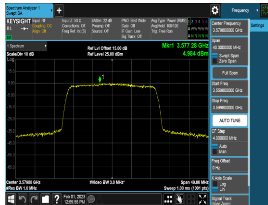
SCC_20M_3579.8MHz_QPSK_FULLLRB_PSD
