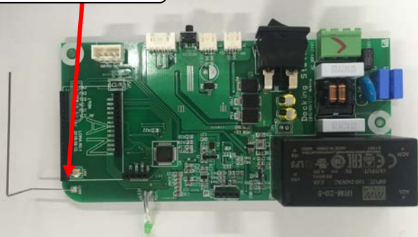
Lora Antenna
