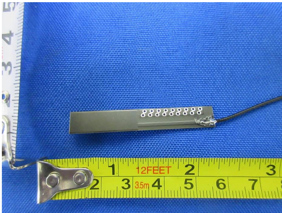
Antenna-3
