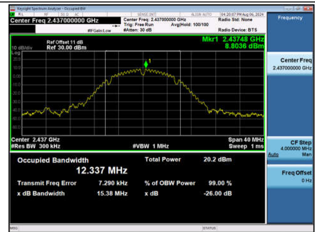
11B-Ant1-2437
