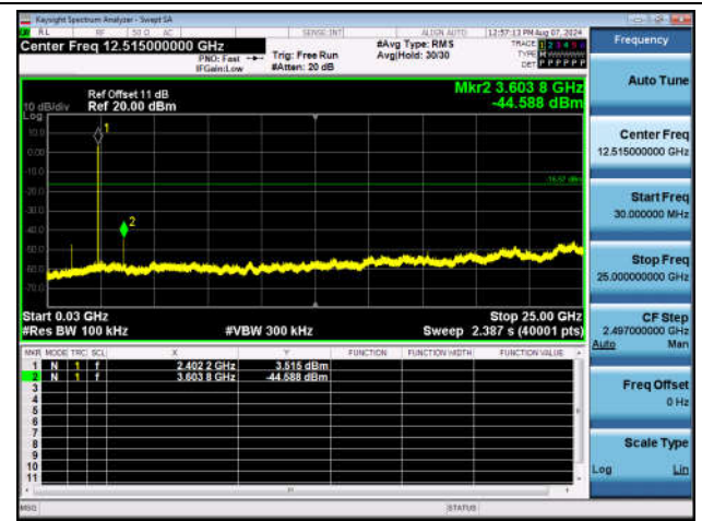
BLE_2M-Ant1-2402-30~25000-PASS
