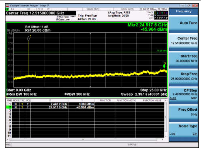
BLE_2M-Ant1-2440-30~25000-PASS
