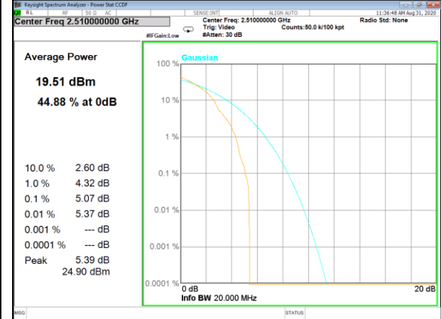
Band7_1_Q16_Low
