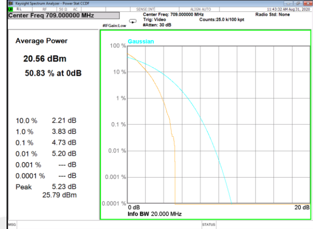
Band17_50_Q16_Low
