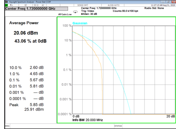
Band4_1_Q16_Low
