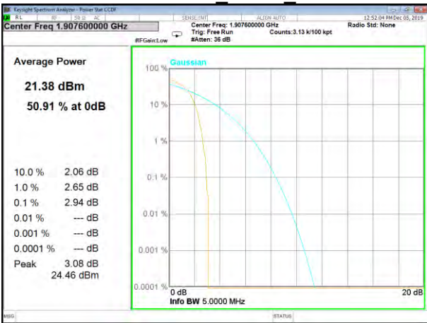
HSUPA2_Higher_
