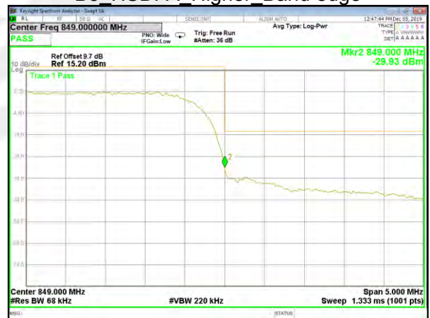
B5_HSUPA_Higher_Band edge
